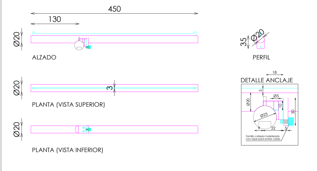
DETALLE FRONTALES EXTRAIBLES
