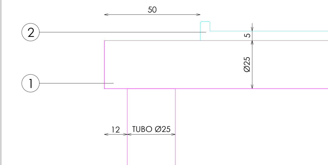
DETALLE A
