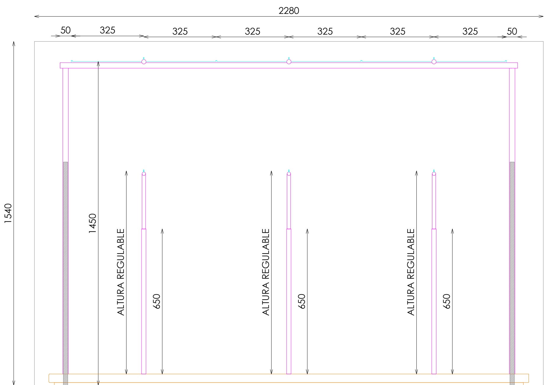
ALZADO FRONTAL
