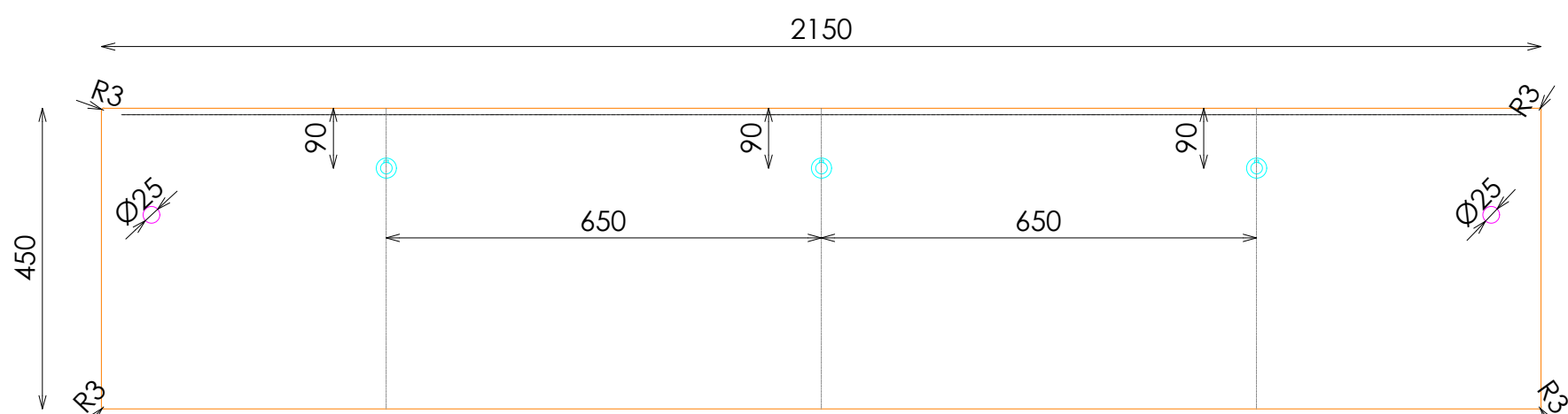
PLANTA TARIMA
