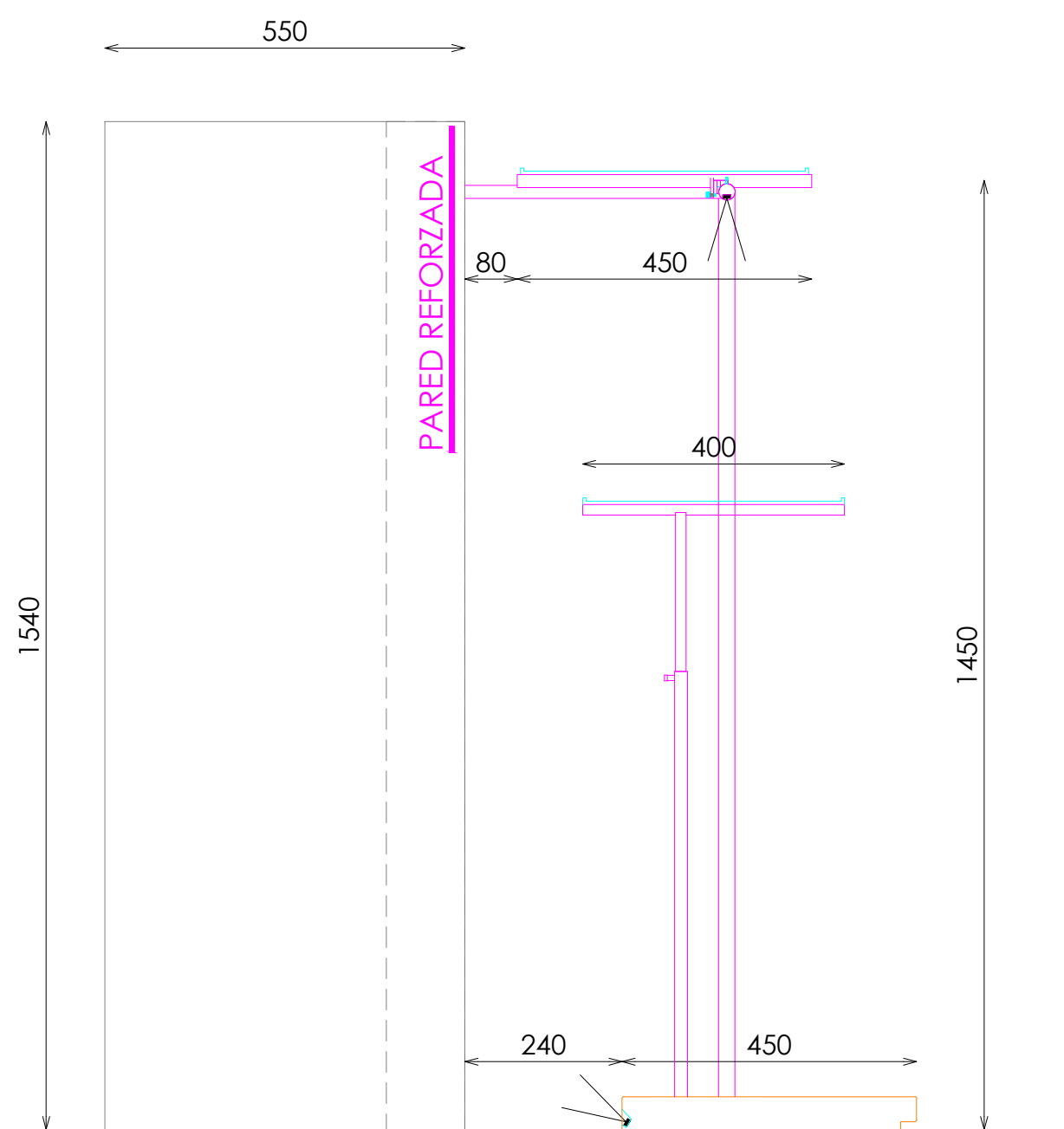
SECCIÓN
