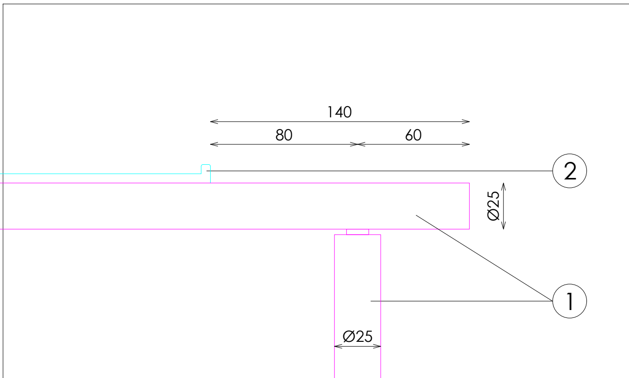
DETALLE A
