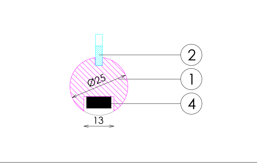
DETALLE B
