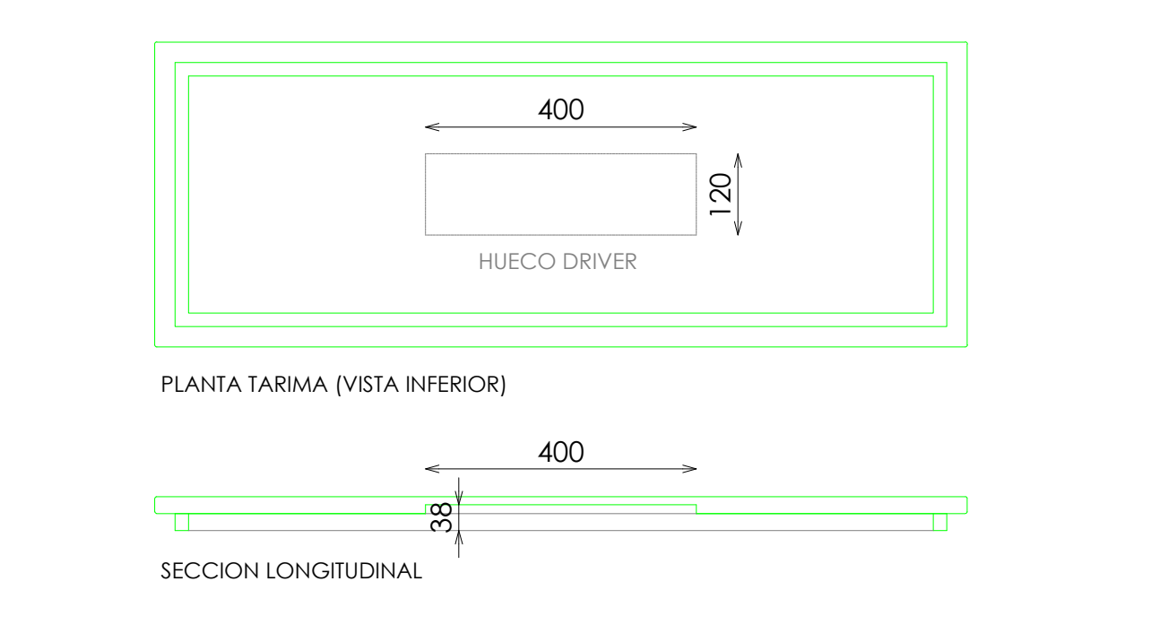
DETALLE TARIMA. HUECO DRIVER
