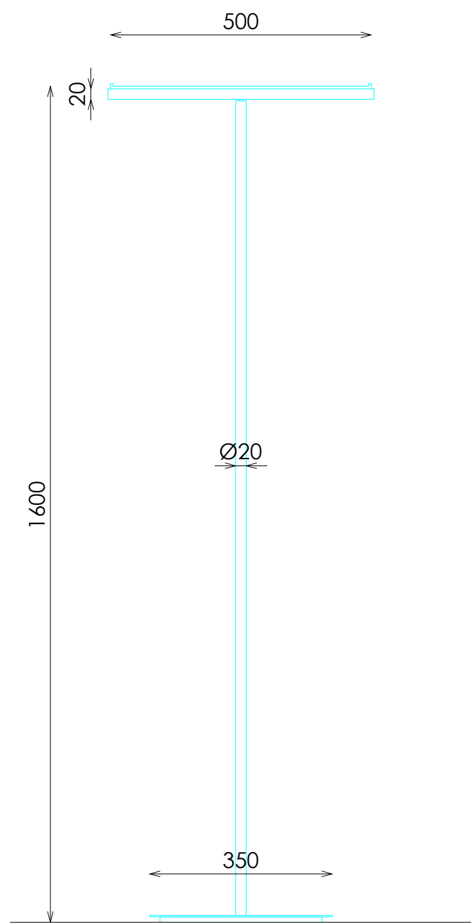
ALZADO
