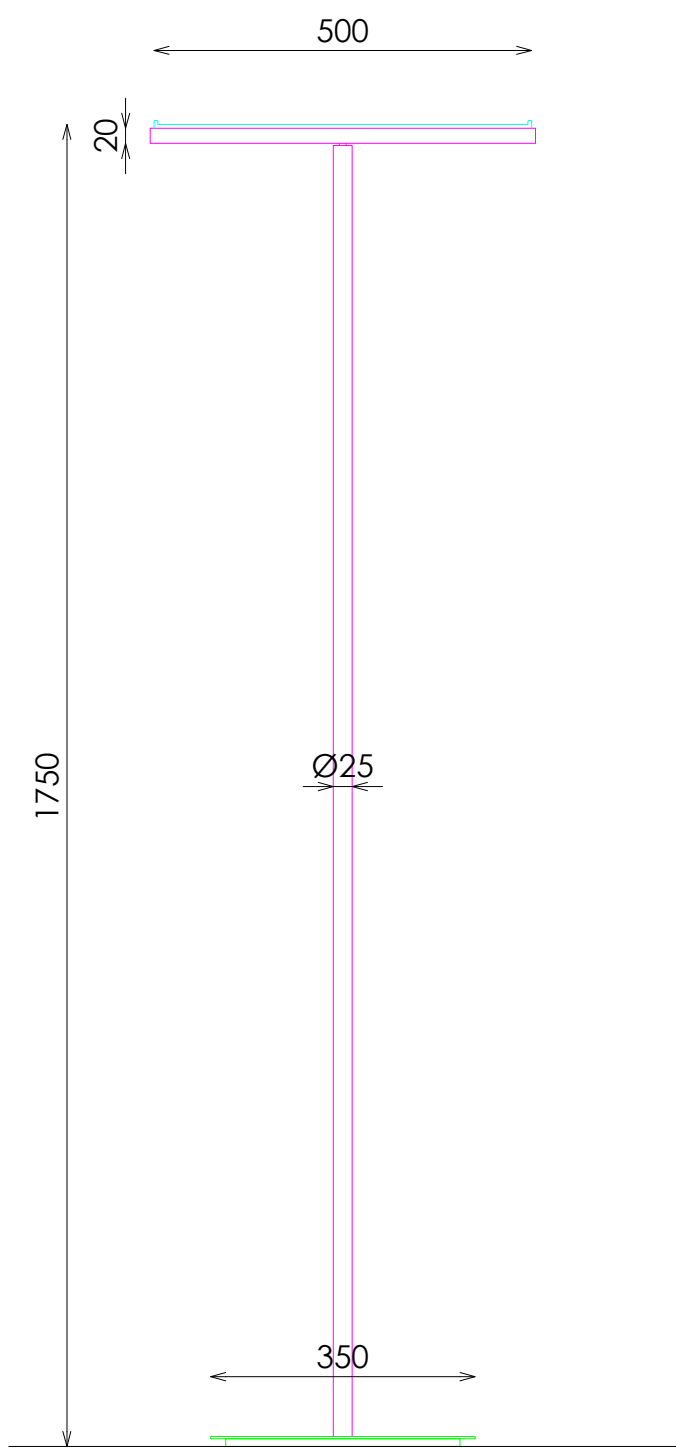
ALZADO
