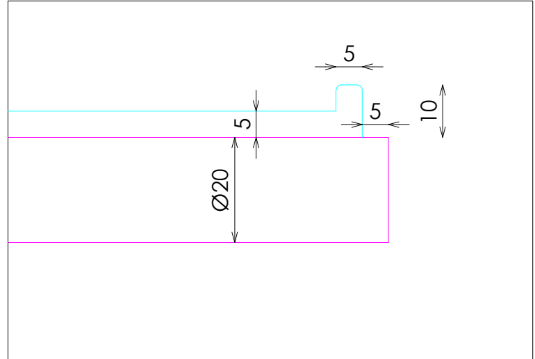
DETALLE C
