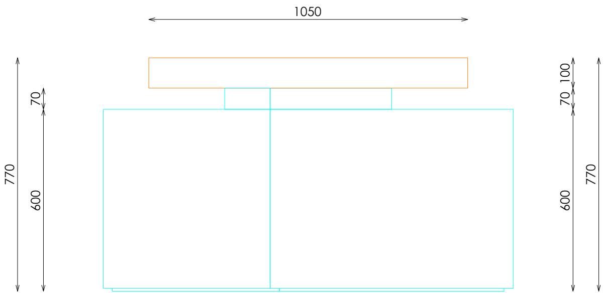
ALZADO LATERAL
