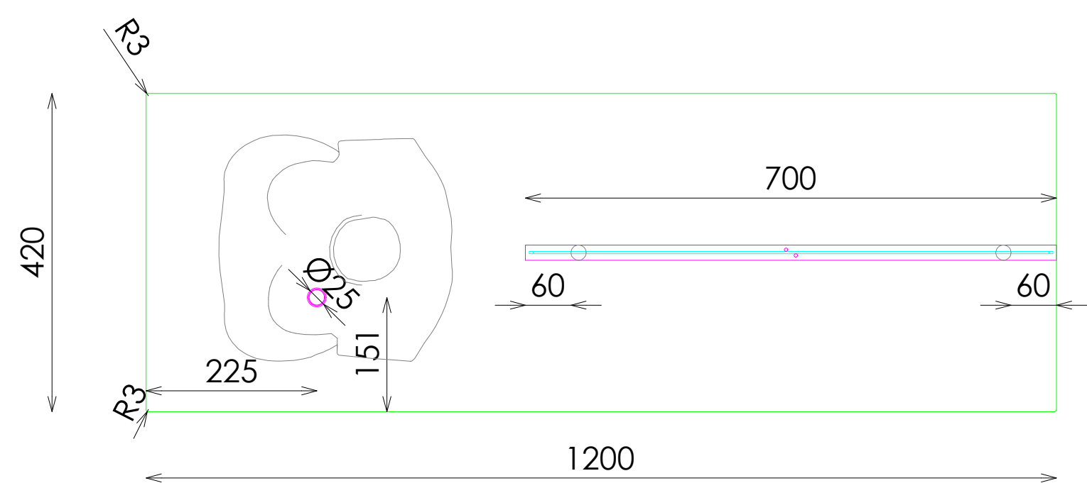
PLANTA
