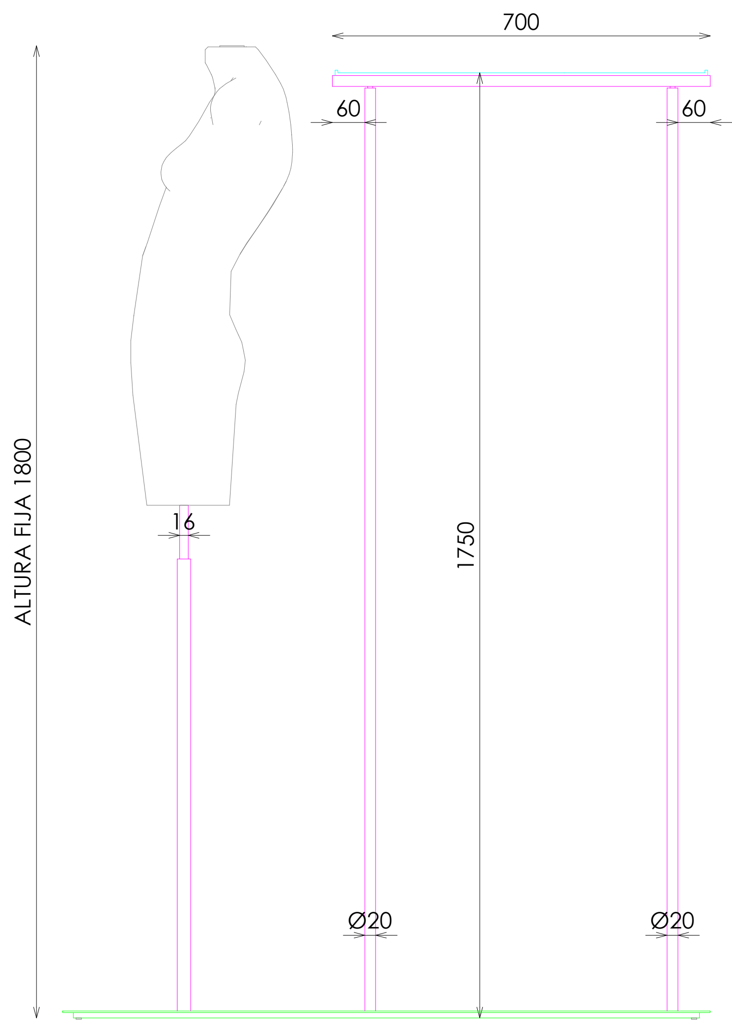
ALZADO LATERAL
