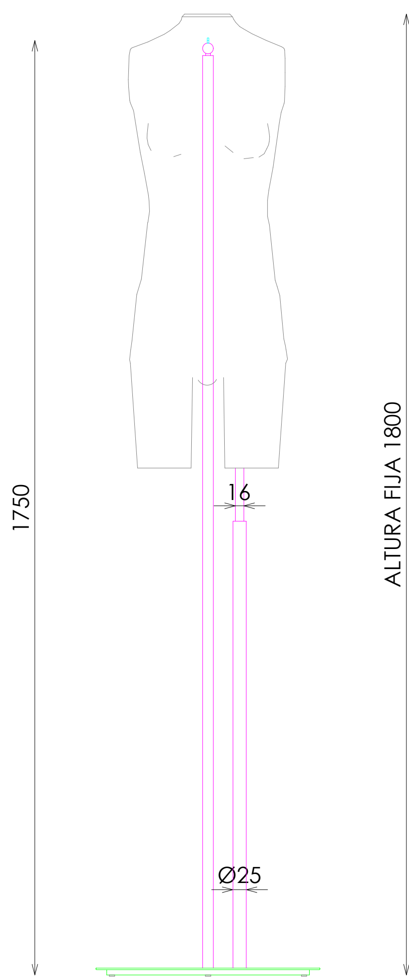
ALZADO FRONTAL
