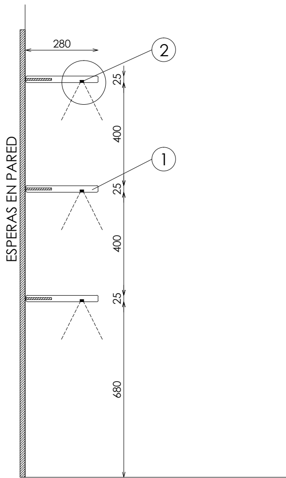
SECCION
