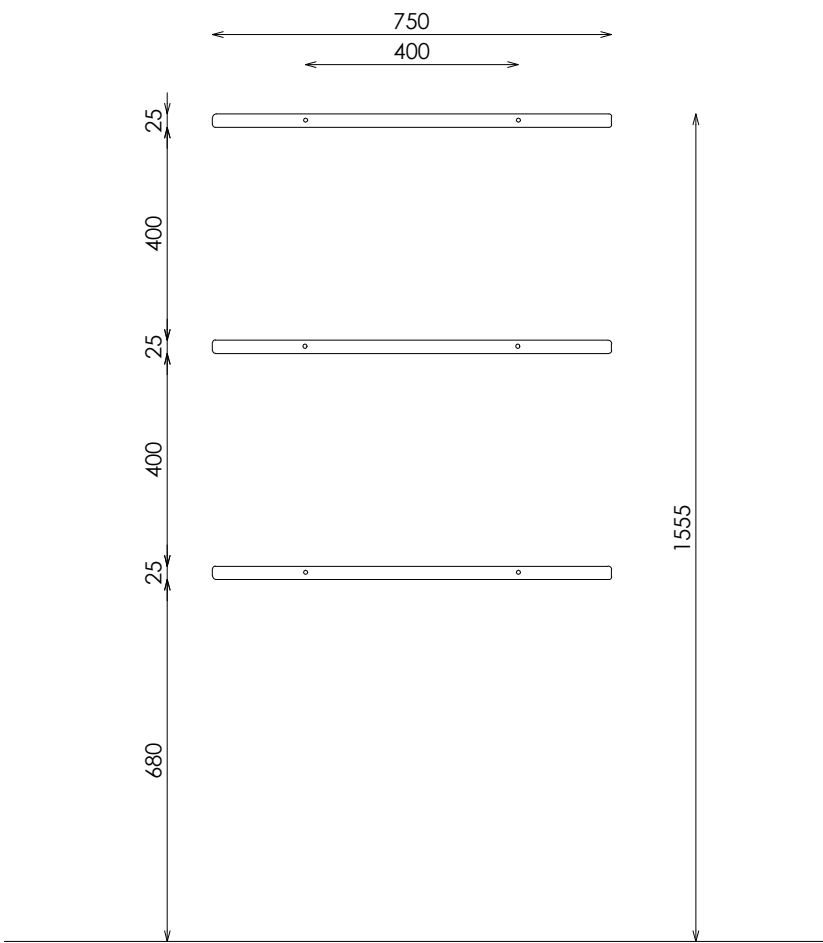
ALZADO
