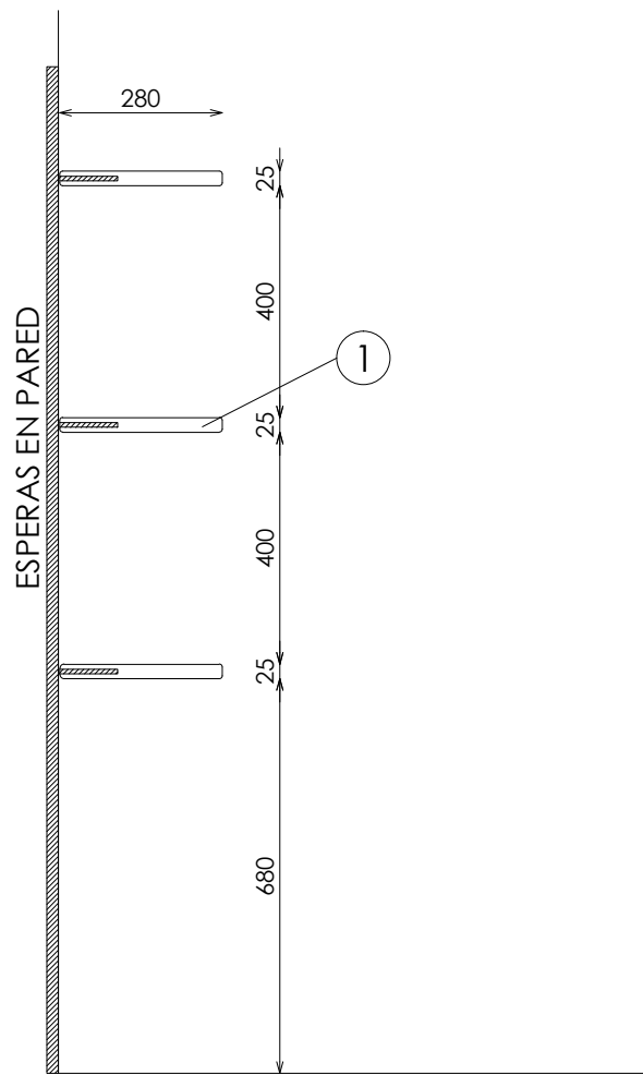
ALZADO LATERAL
