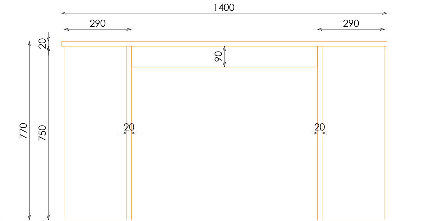
ALZADO FRONTAL
