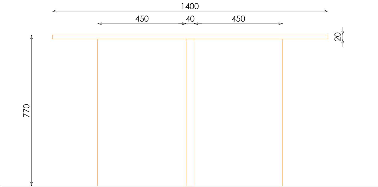
ALZADO LATERAL
