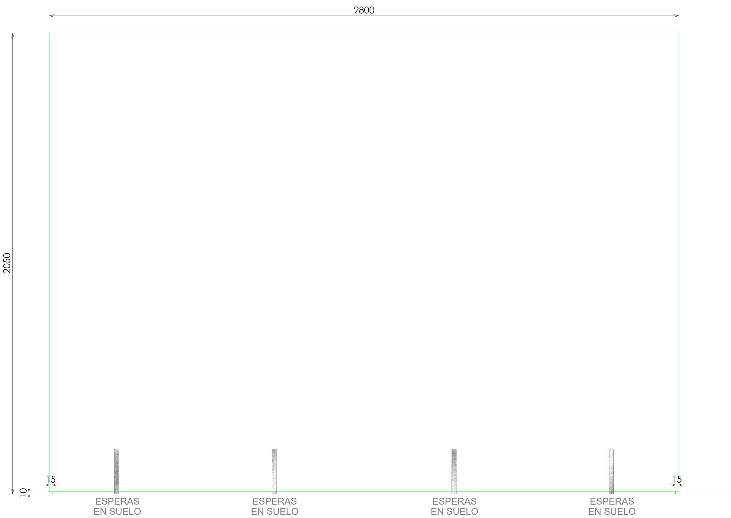
ALZADO
