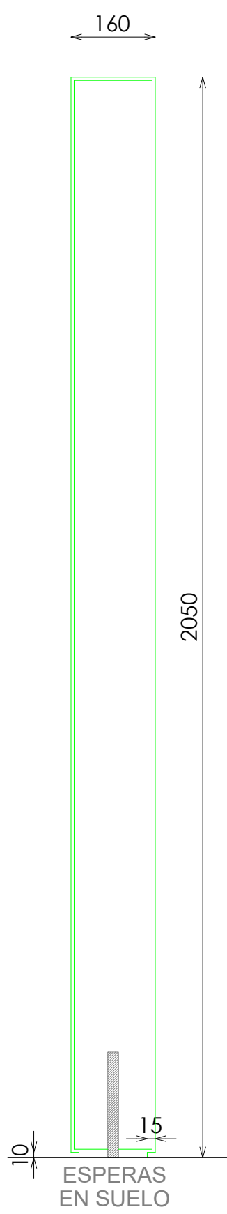
SECCION
