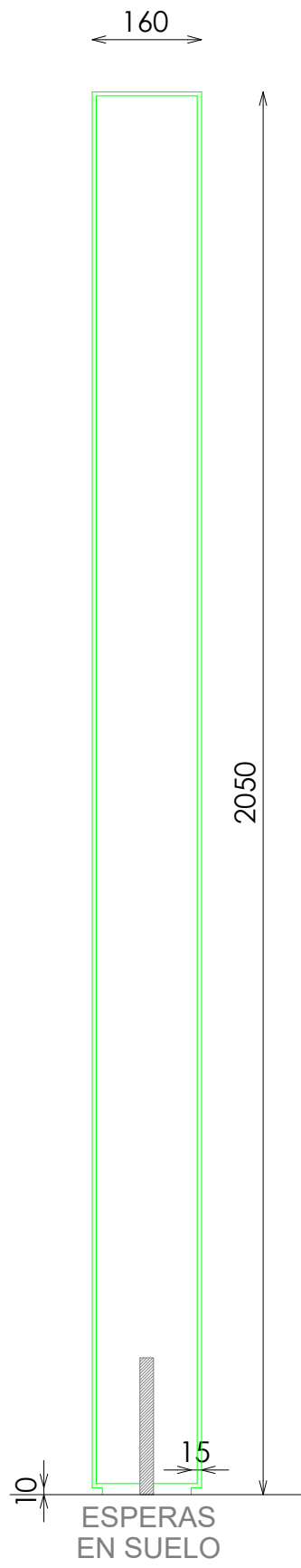
SECCION
