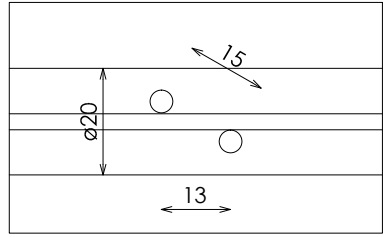
DETALLE C
