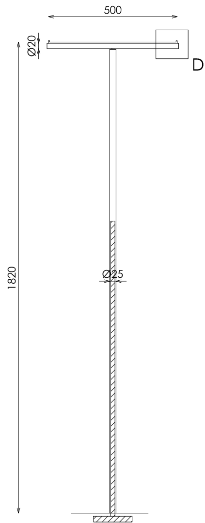
ESPERAS EN SUELO ALZADO
