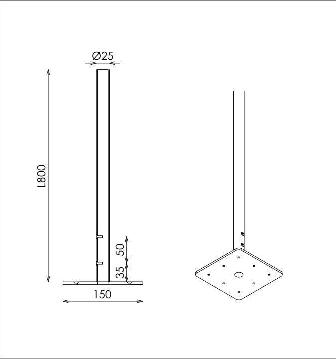
DETALLE ESPERAS SUELO
