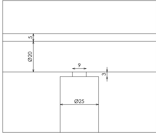
DETALLE A
