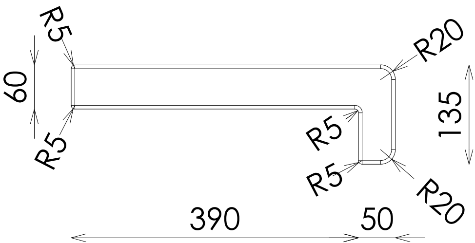
ALZADO LATERAL
