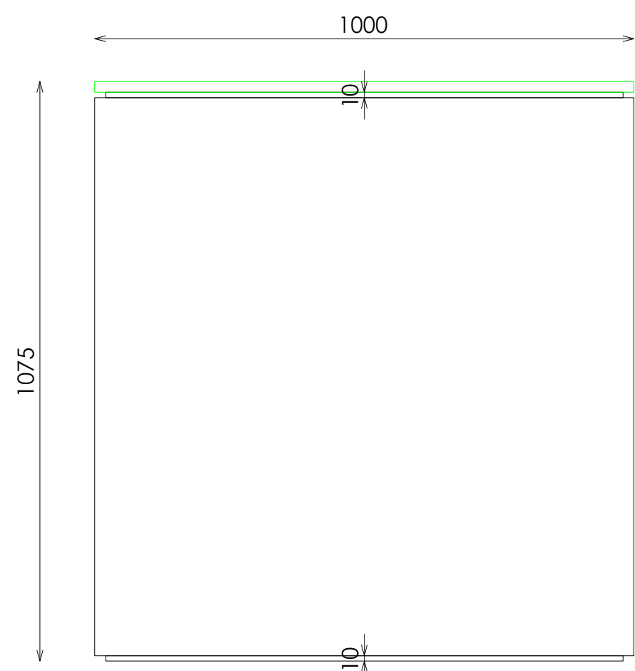
ALZADO FRONTAL
