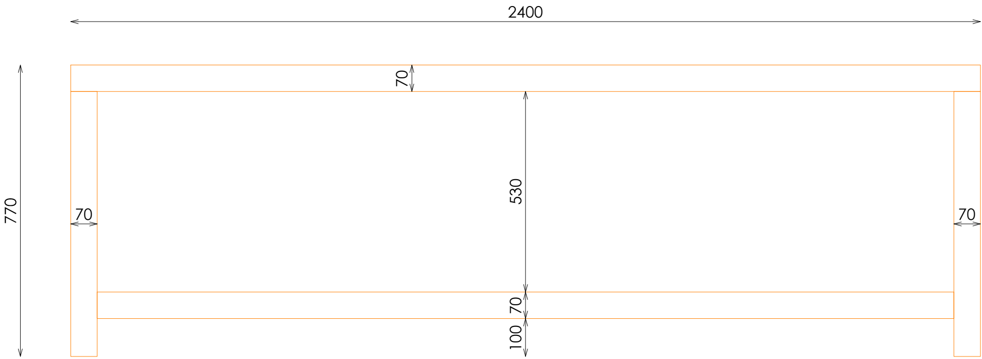
ALZADO
