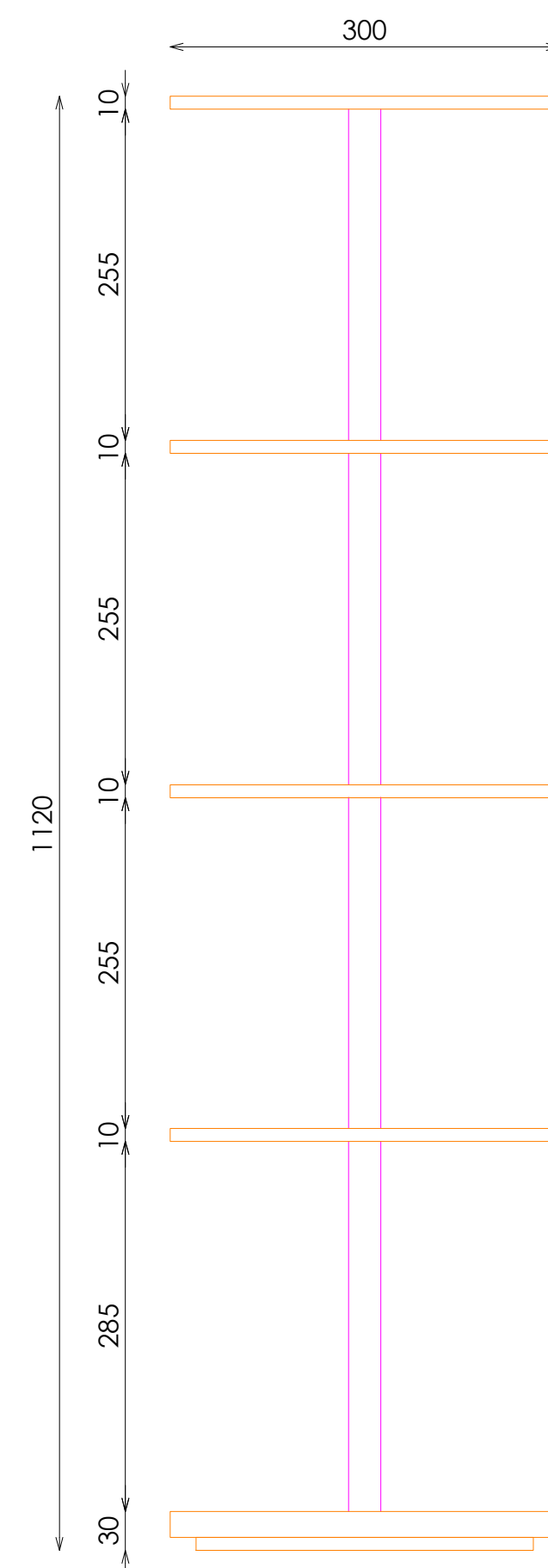
ALZADO
