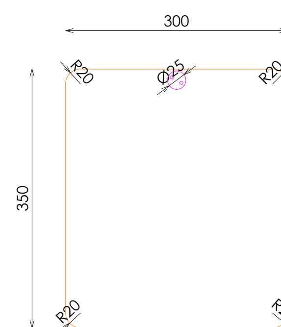
PLANTA
