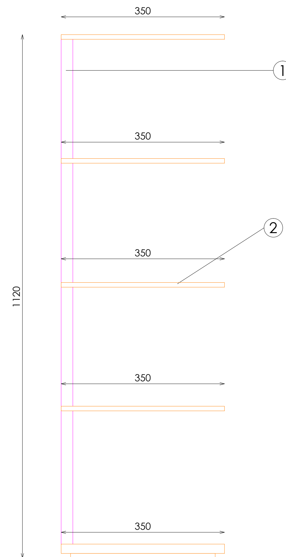
ALZADO LATERAL
