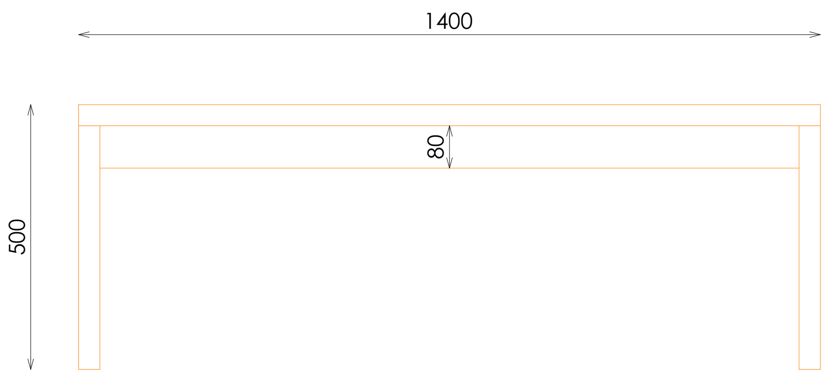
ALZADO
