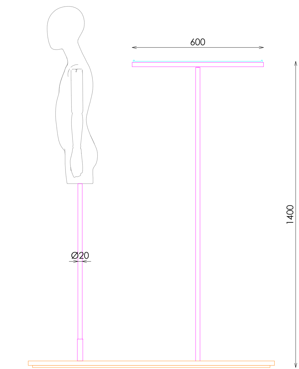
ALZADO
