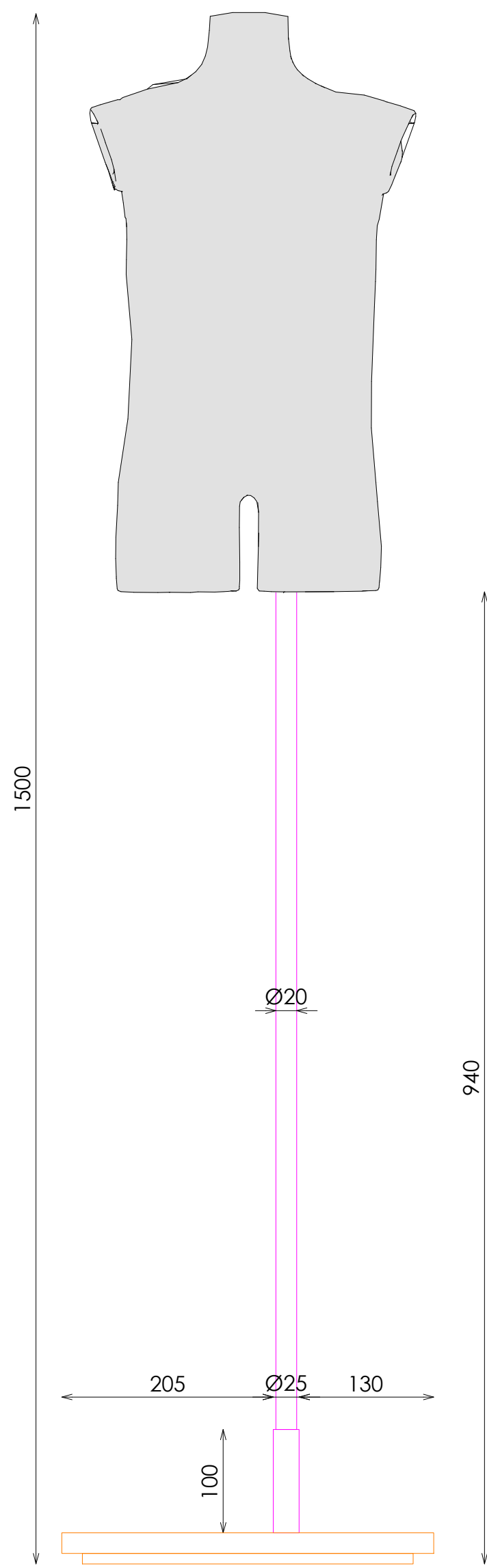
ALZADO FRONTAL
