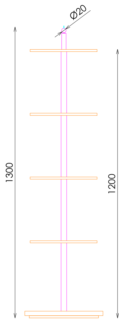
PERFIL
