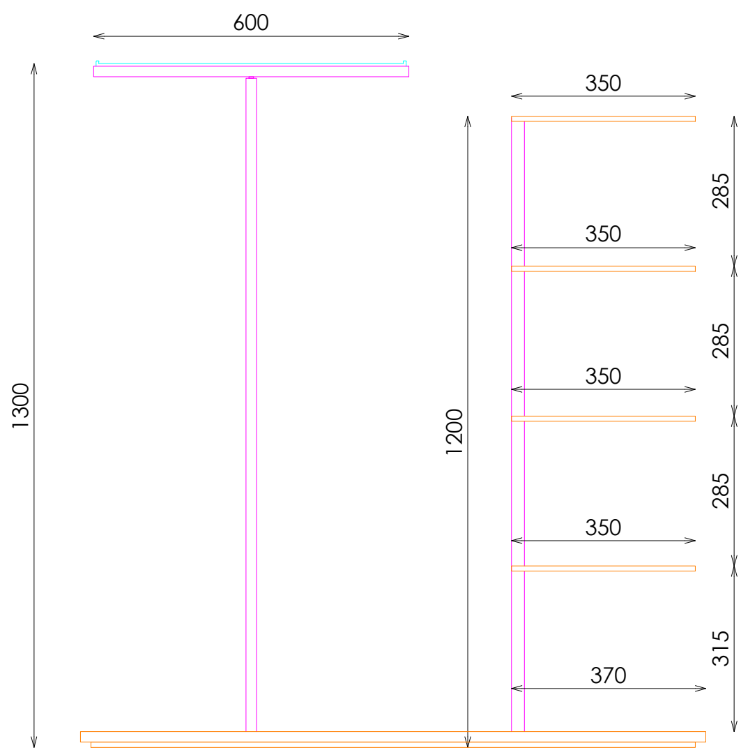
ALZADO
