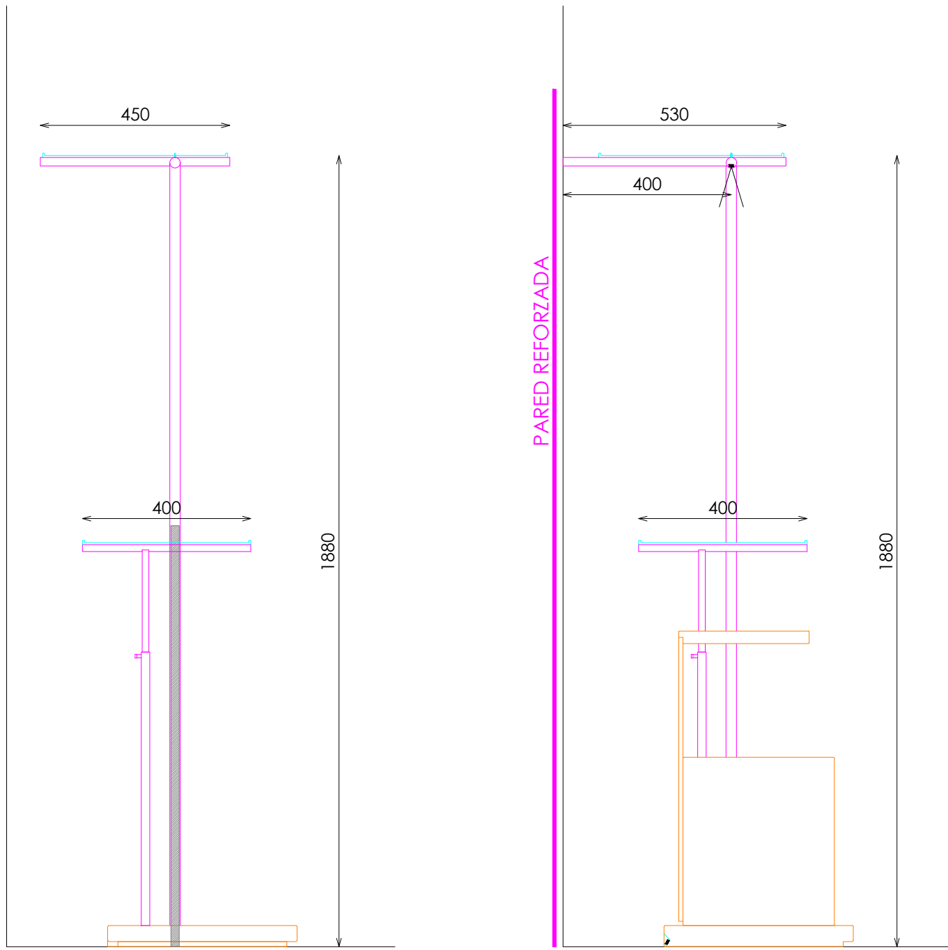
ALZADO LATERAL
