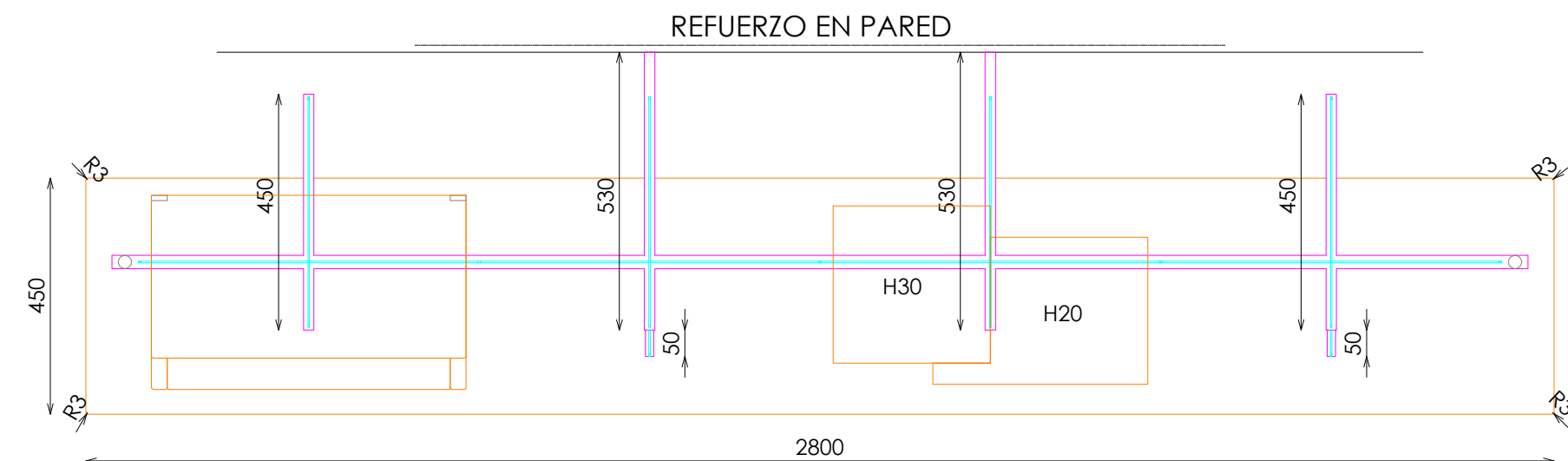
PLANTA
