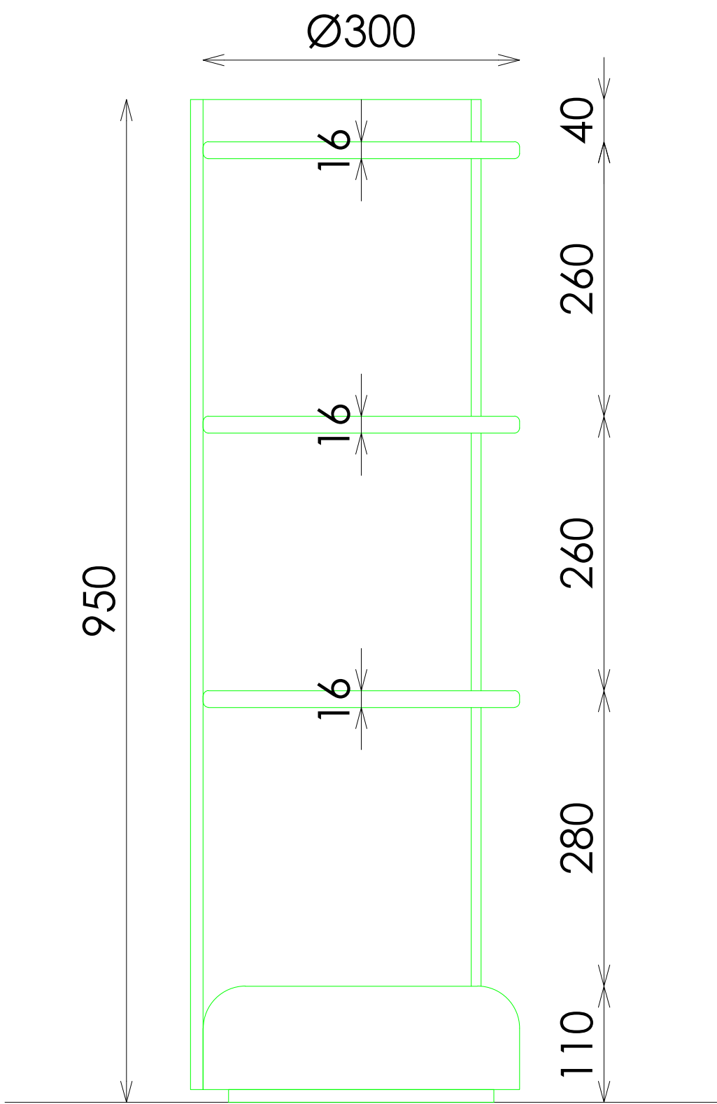
ALZADO
