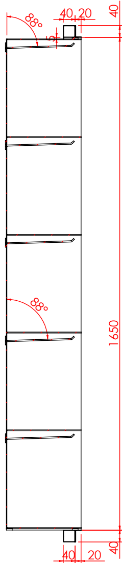
剖面 AG-AG
