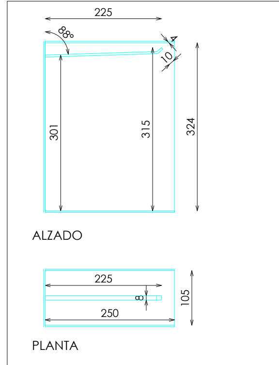
DET. PINCHO FIJO
