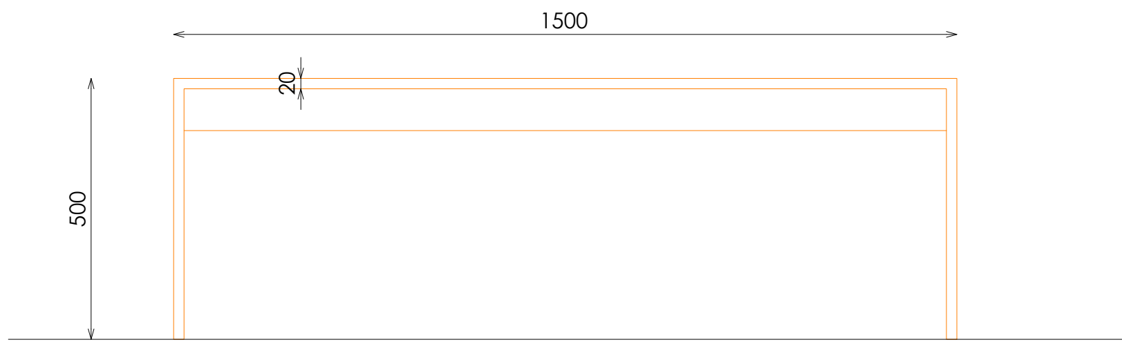
ALZADO FRONTAL
