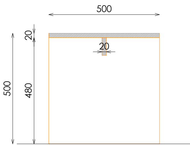
SECCIÓN
