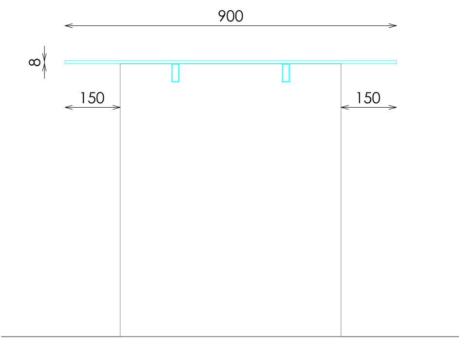
SECCIÓN
