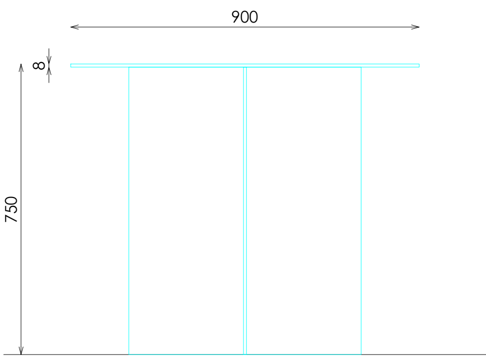
ALZADO LATERAL
