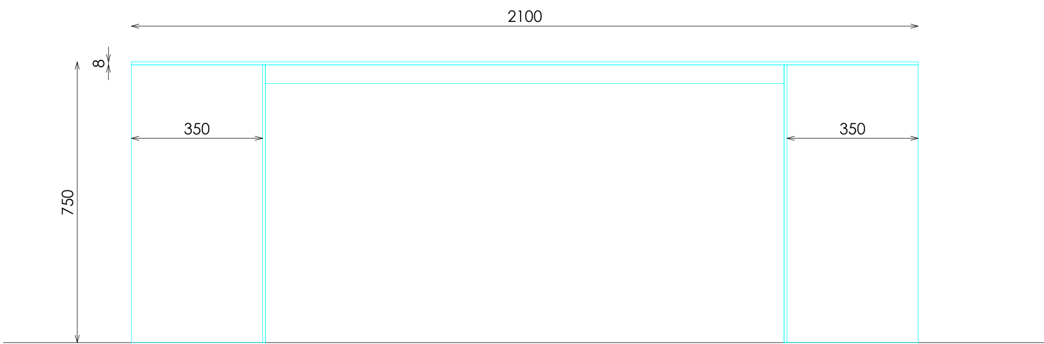
ALZADO FRONTAL
