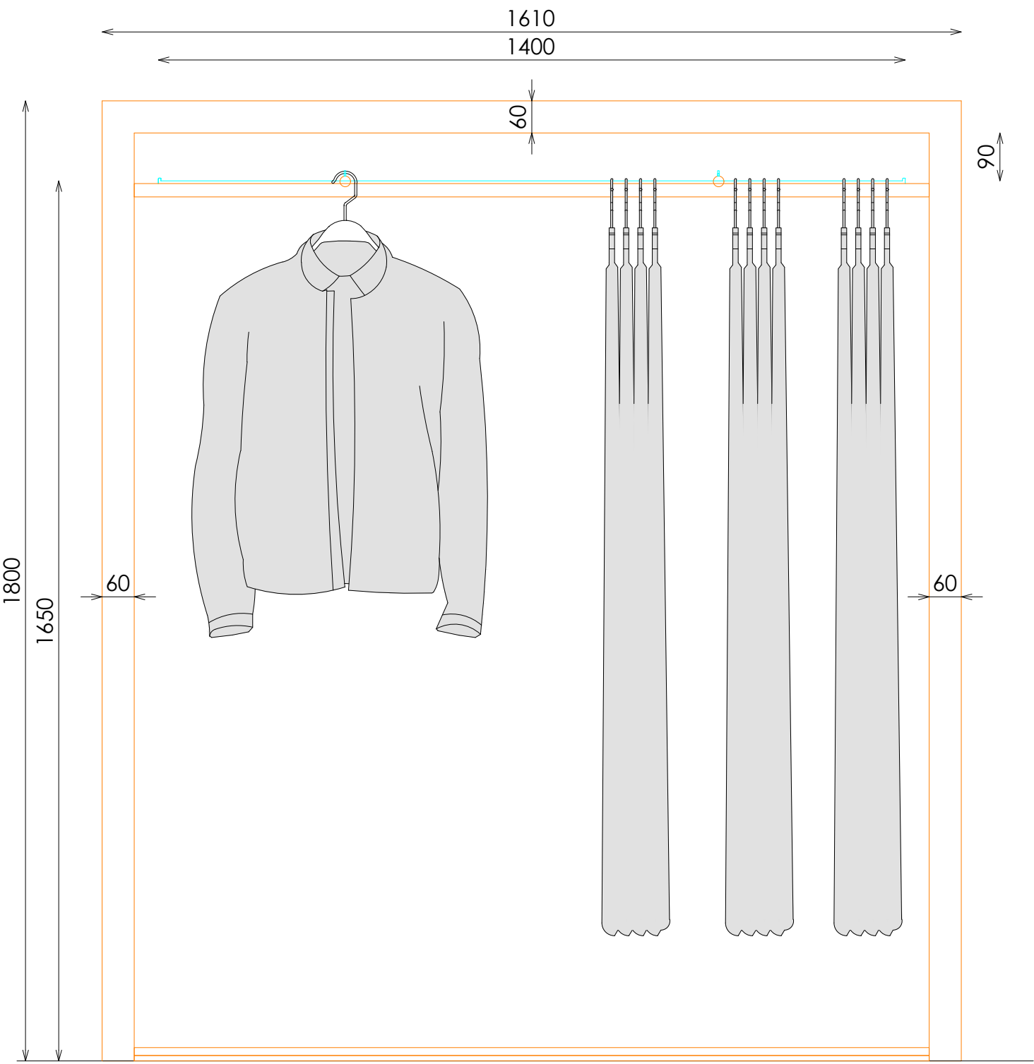
ALZADO
