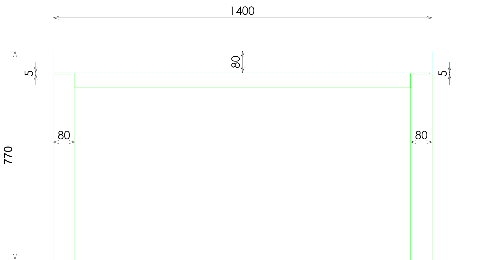
ALZADO FRONTAL
