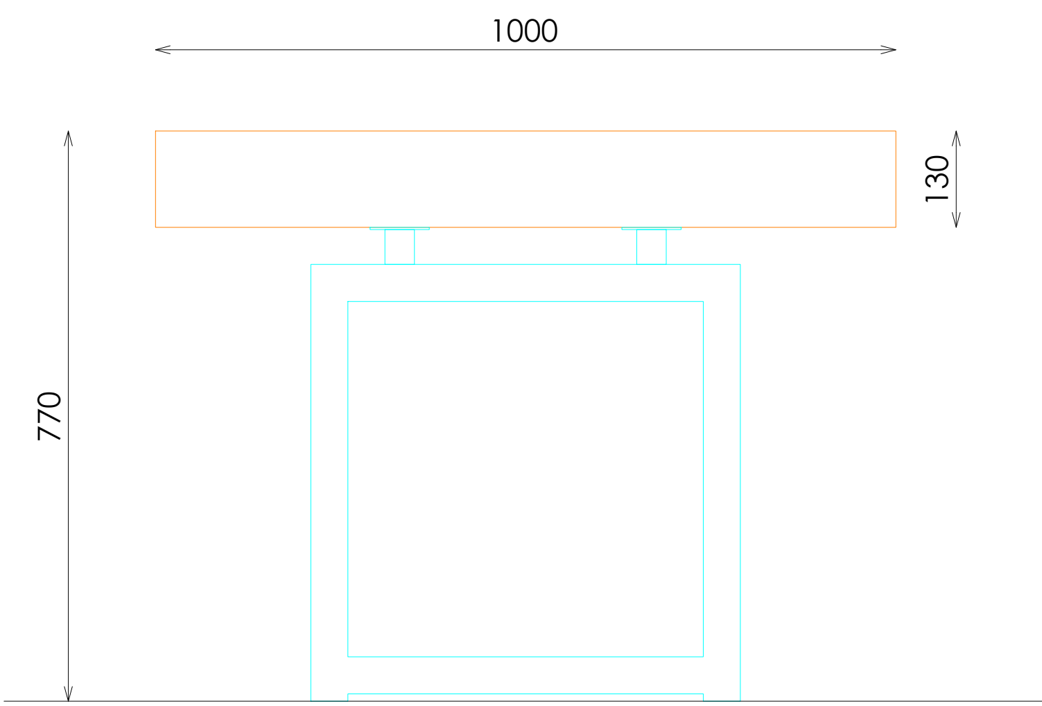
ALZADO LATERAL
