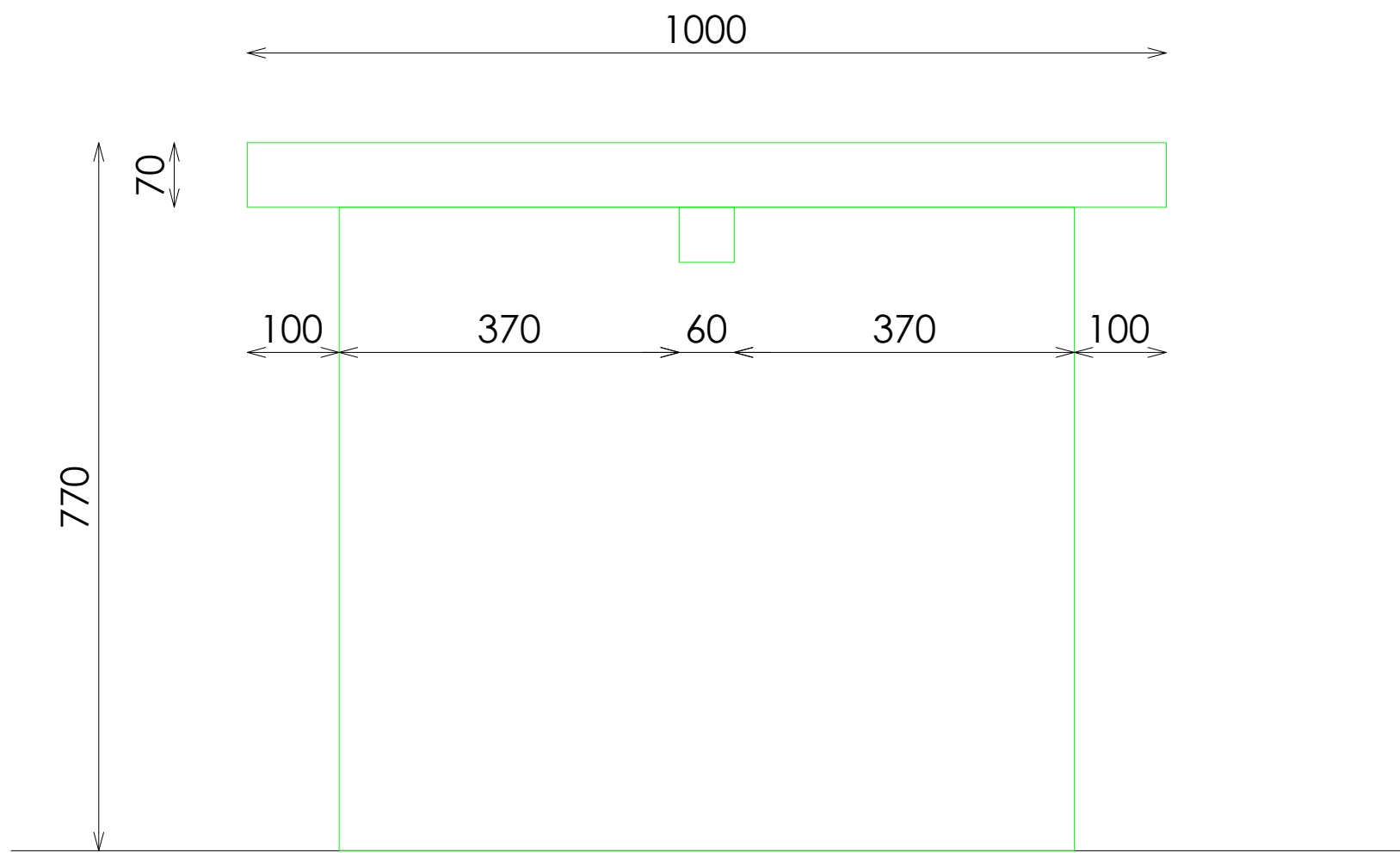
SECCION LATERAL
