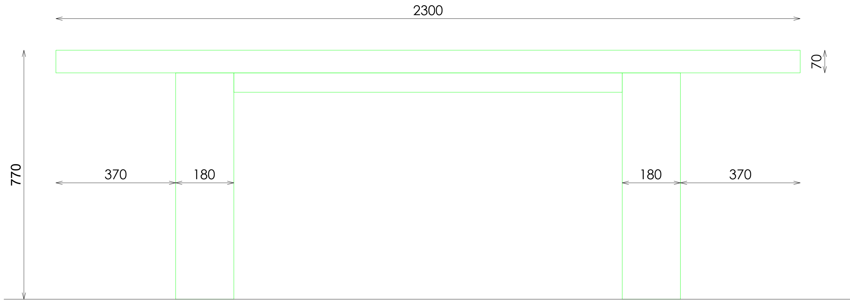
ALZADO FRONTAL
