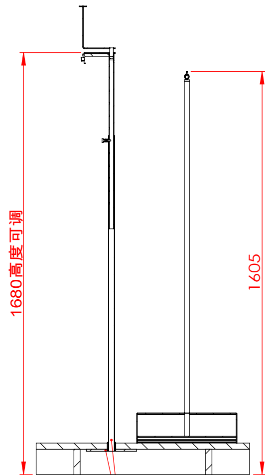
剖面 A-A
