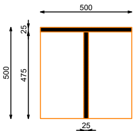
SECCIÓN
