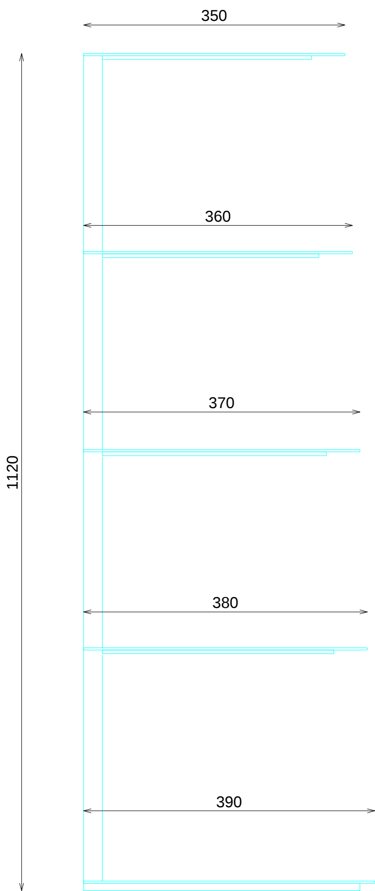
ALZADO LATERAL
