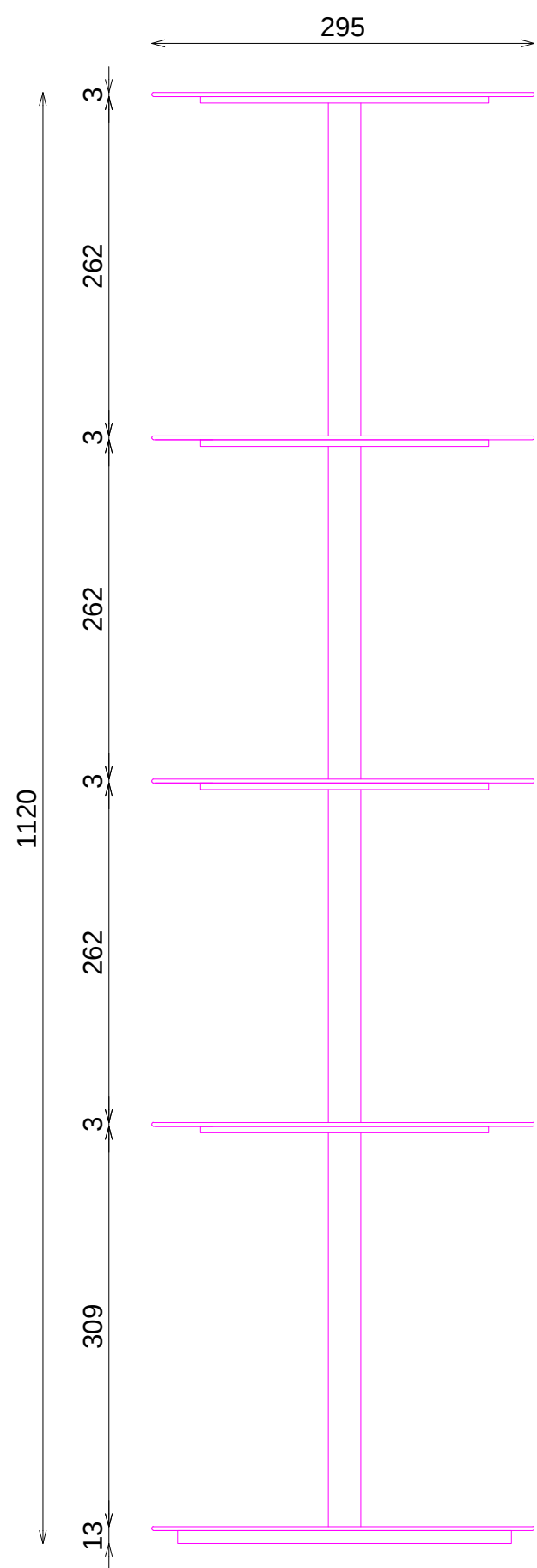
ALZADO
