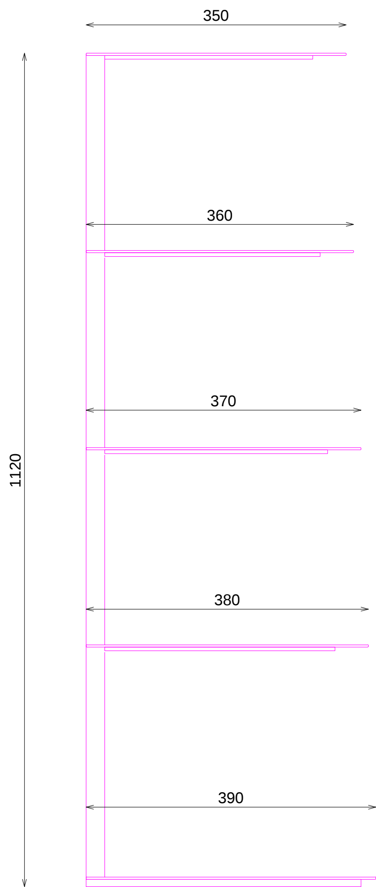
ALZADO LATERAL
