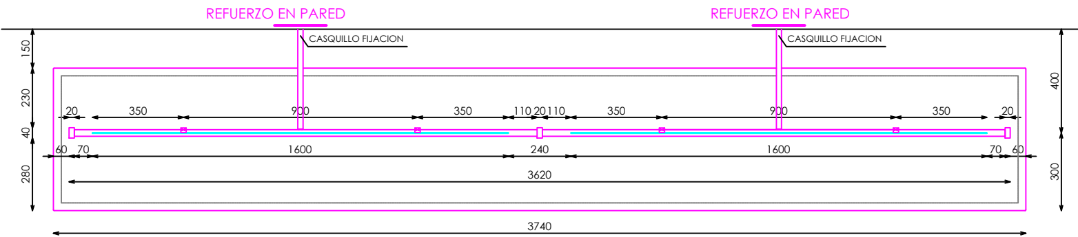
PLANTA
