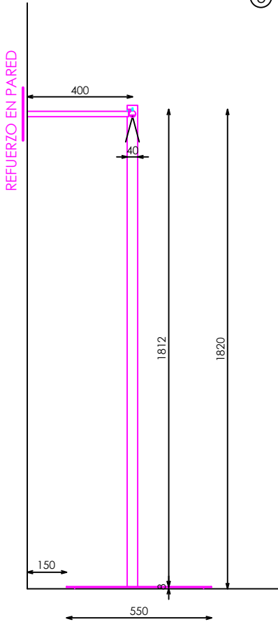
PERFIL SECCIONADO
