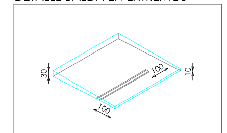
DETALLE BARRA
