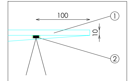
DETALLE BALDA EN EXTREMOS
