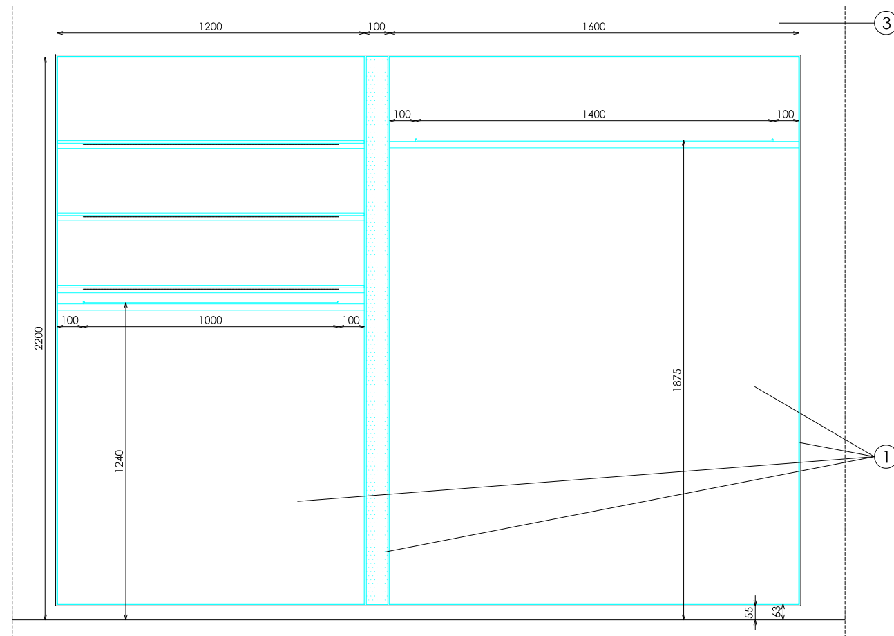
ALZADO
