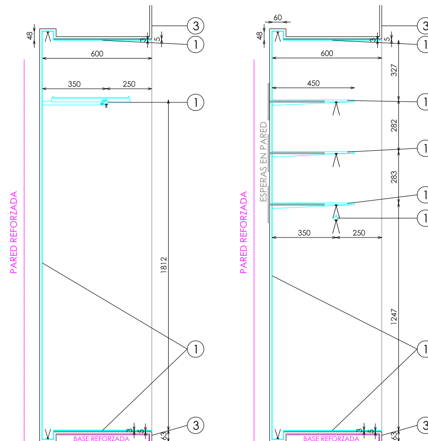
SECCIÓN BARRA
