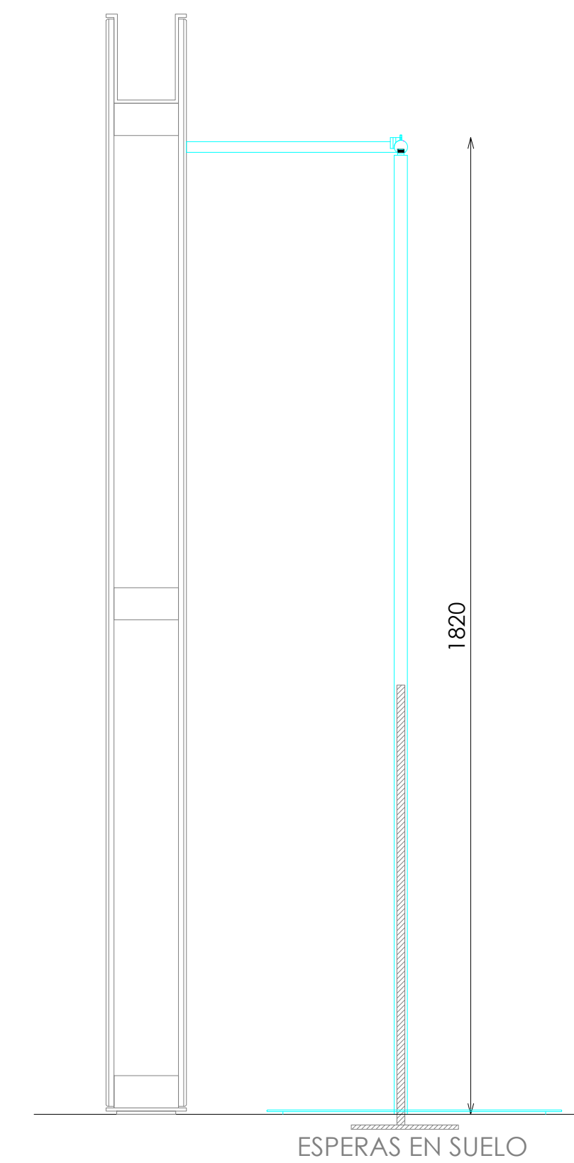
PERFIL
