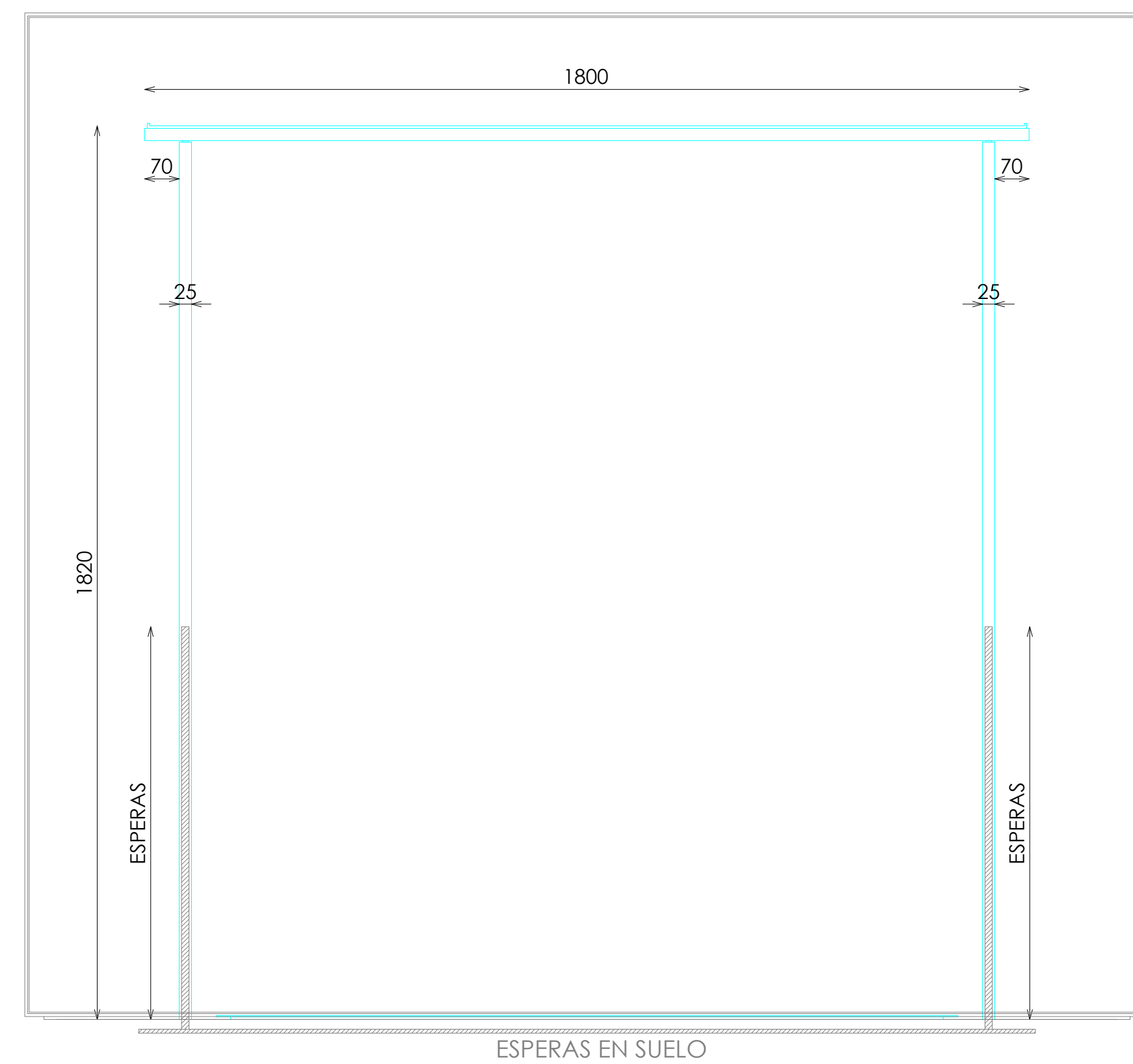
ALZADO
