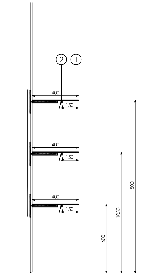
SECCION
