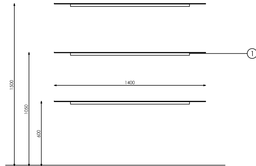
ALZADO
