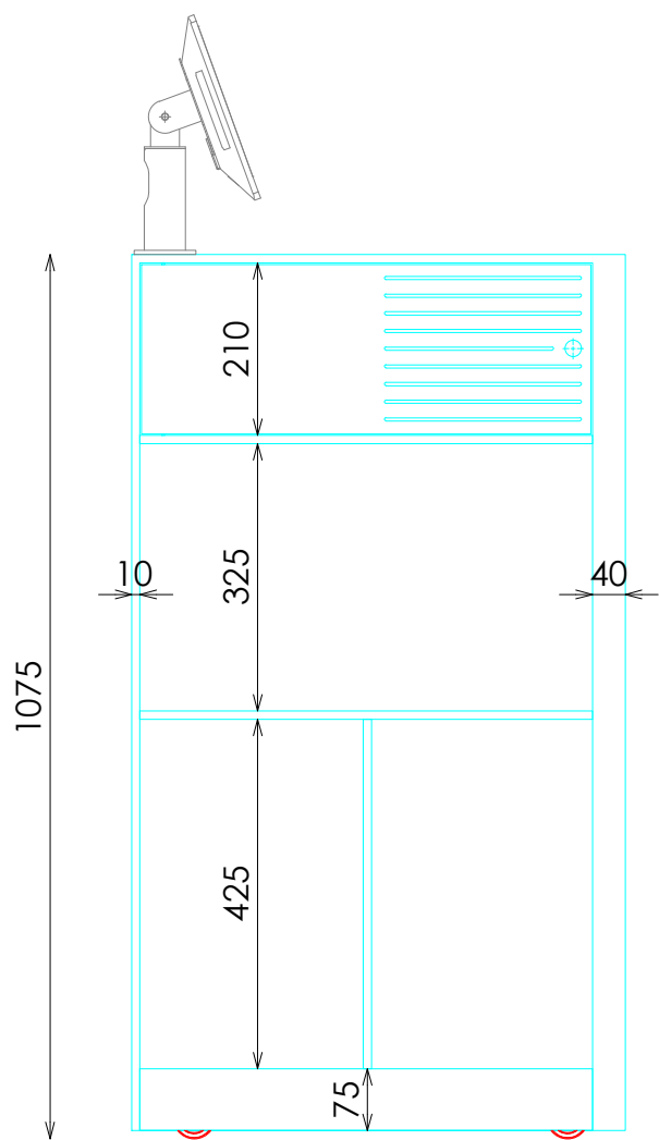
ALZADO TRASERO
