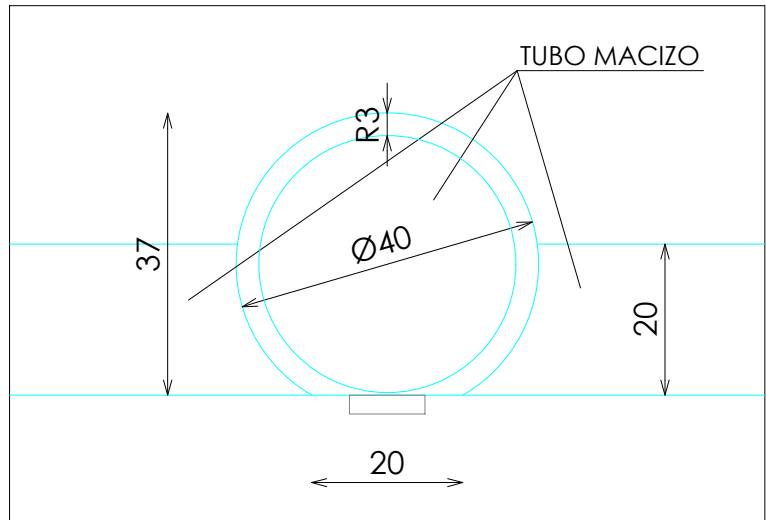
DETALLE D
