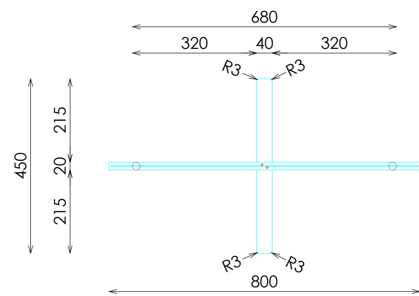
PLANTA
