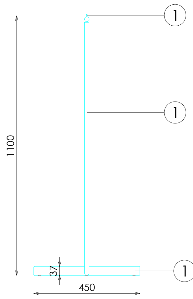
PERFIL
