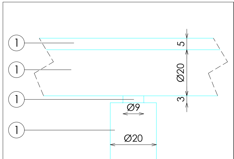
DETALLE A
