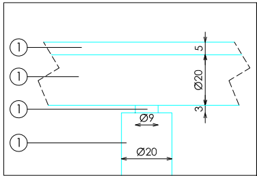
DETALLE A
