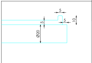
DETALLE C
