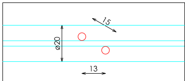
DETALLE C
