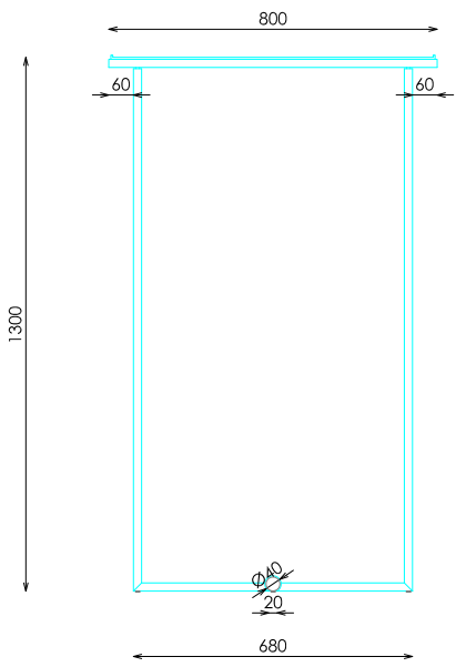
ALZADO
