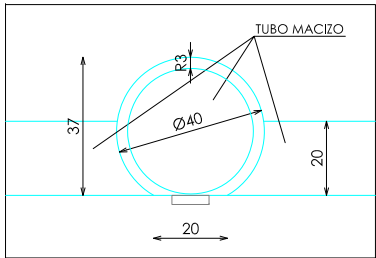
DETALLE D
