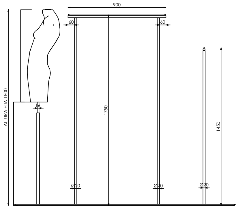
ALZADO LATERAL
