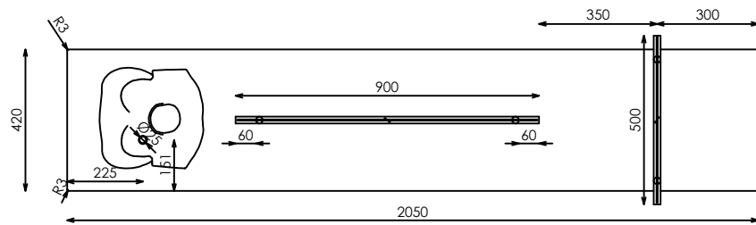
PLANTA
