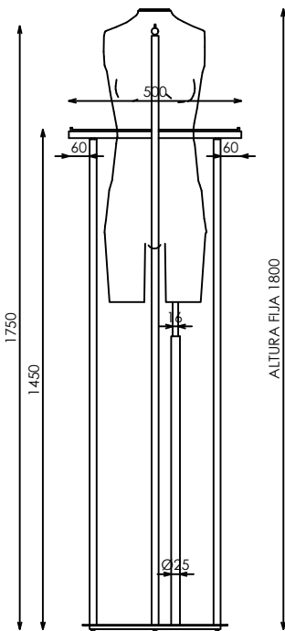
ALZADO FRONTAL
