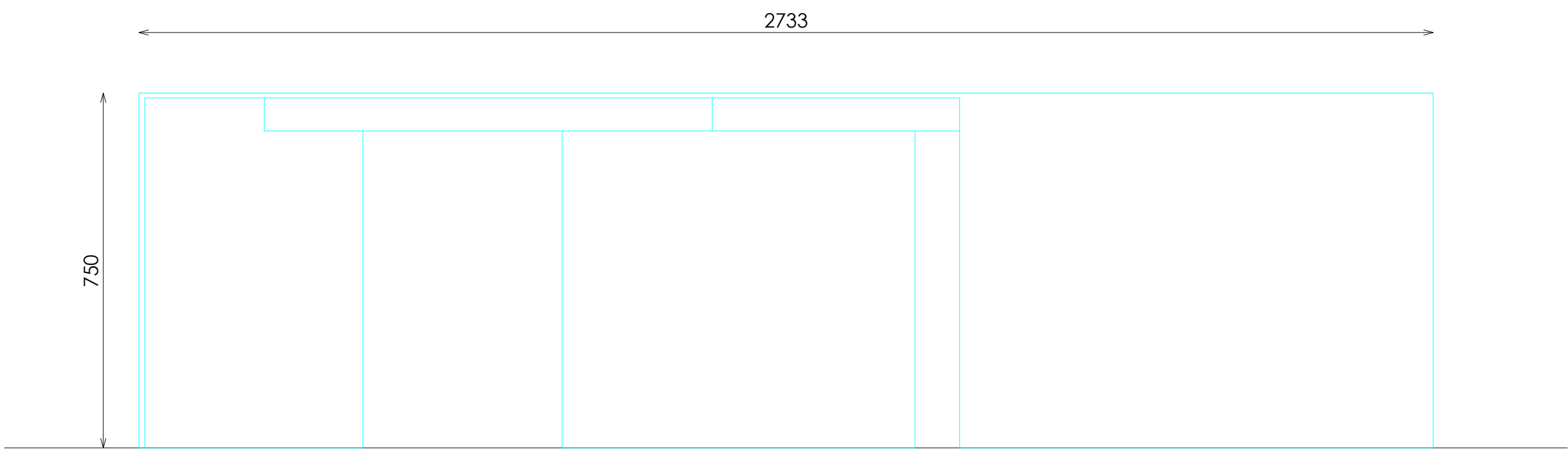
ALZADO FRONTAL
