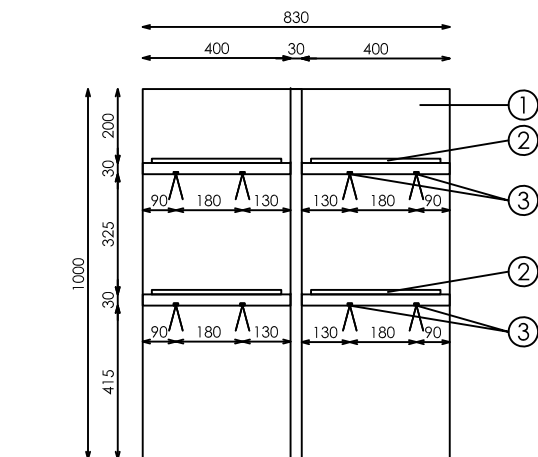
SECCION TRANSVERSAL
