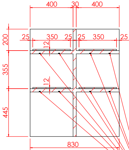
剖面 AG-AG
