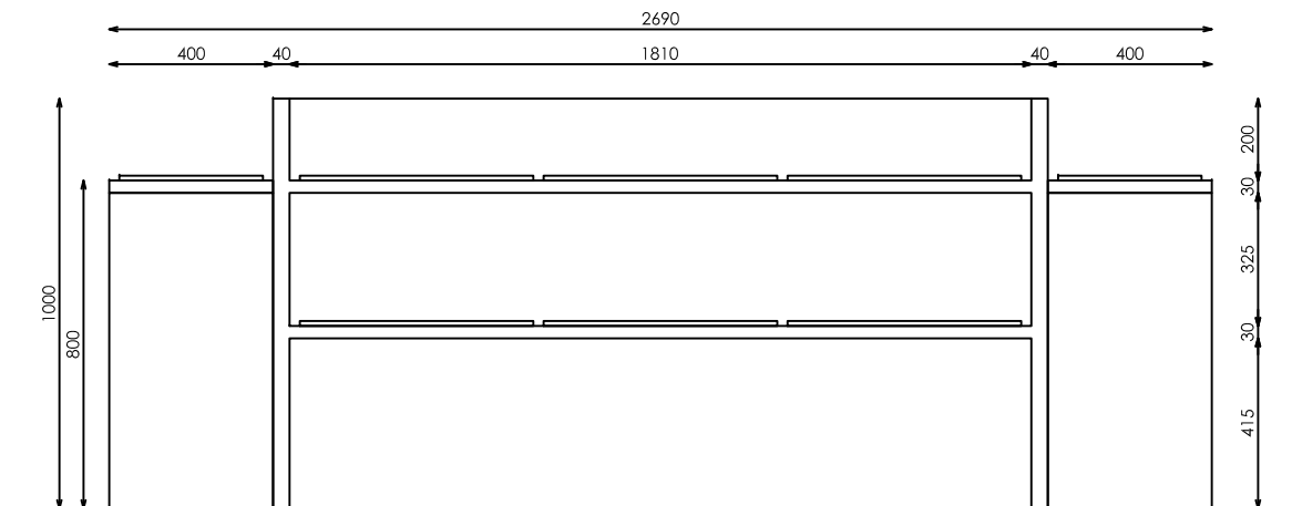
ALZADO FRONTAL
