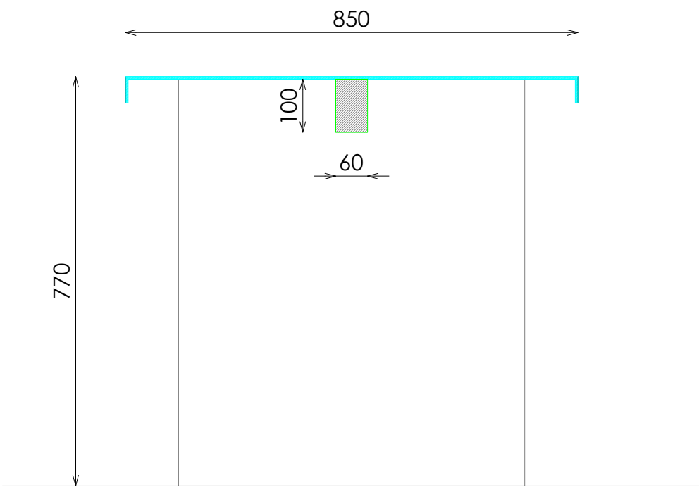
SECCION LATERAL
