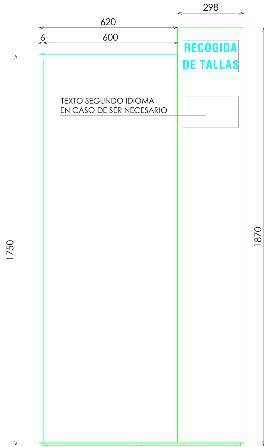
ALZADO POSTERIOR
