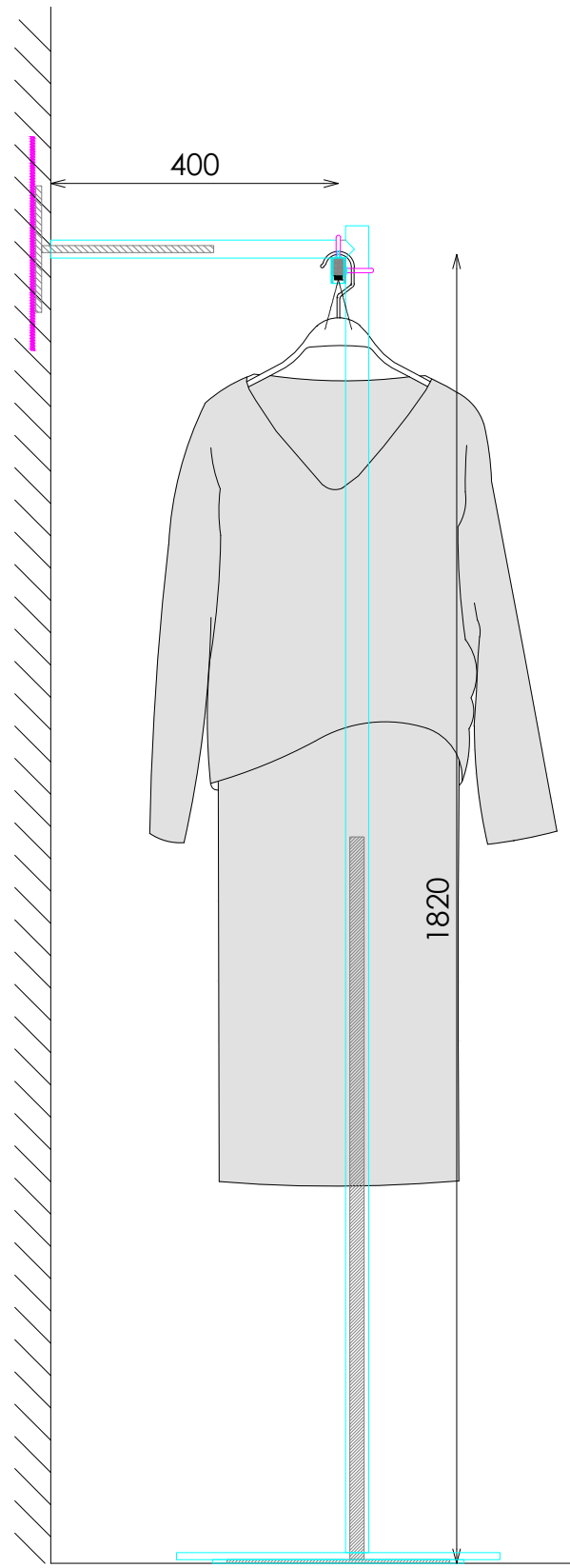
SECCIÓN (ANCLAJE A PARED)
