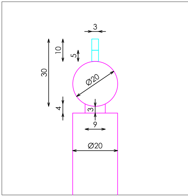
DETALLE B
