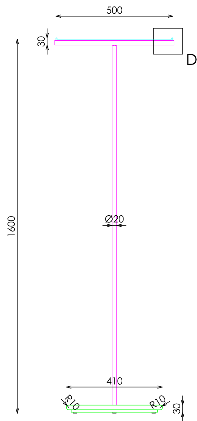
ALZADO
