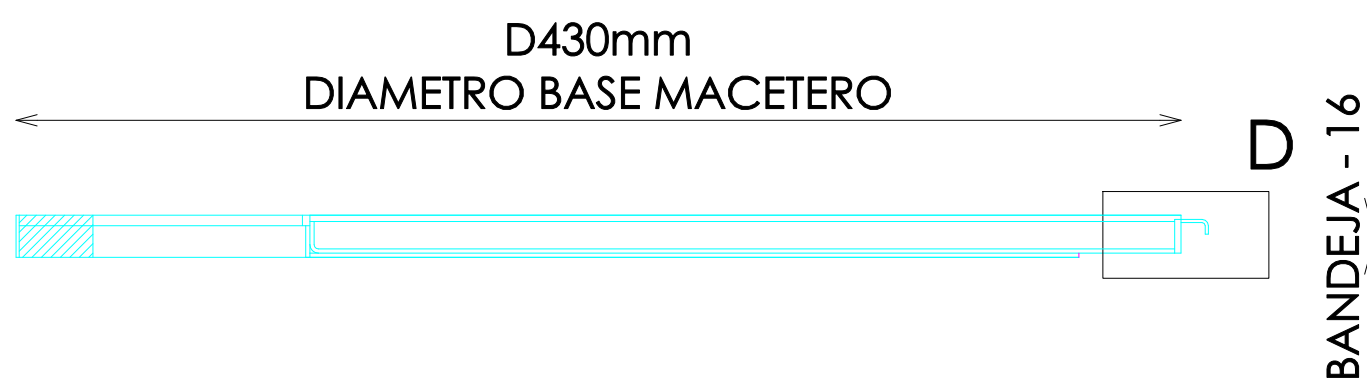
PERFIL SECCIONADO
