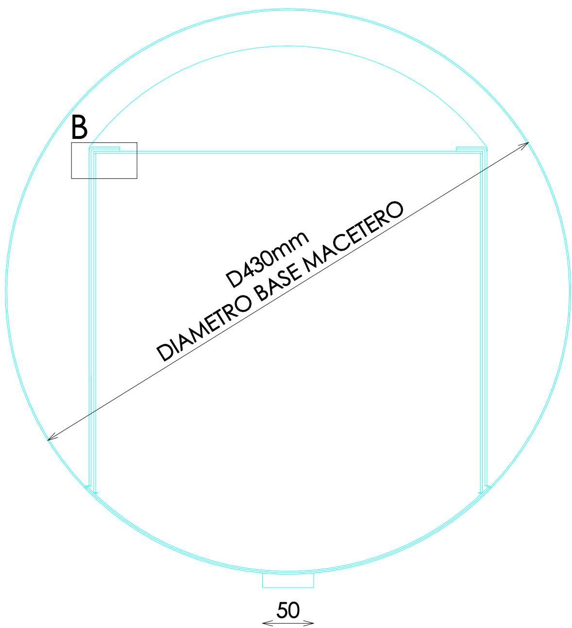
PLANTA SECCIONADA
