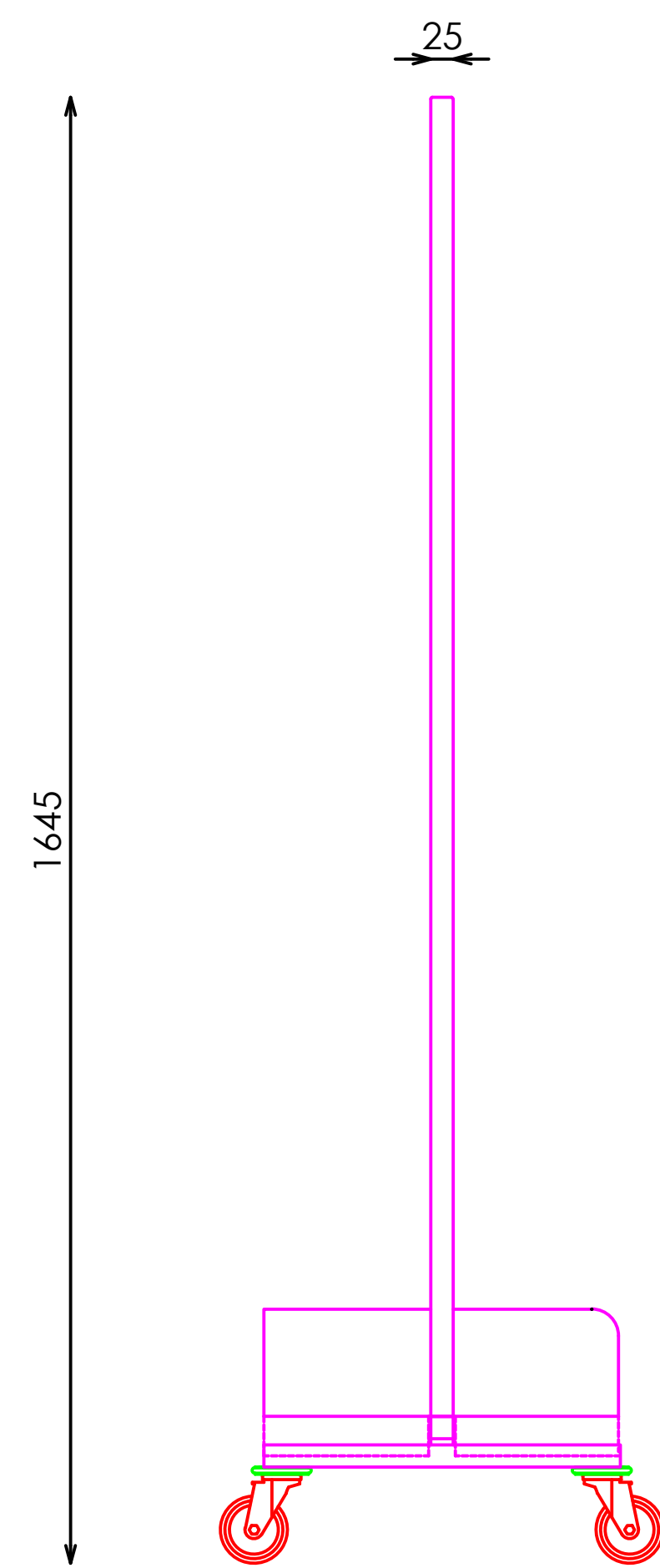
ALZADO LATERAL
