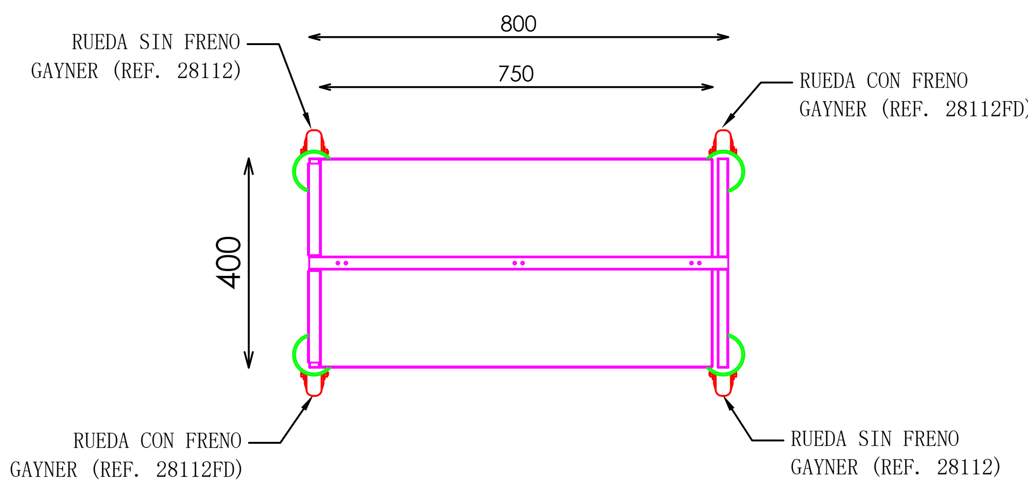
PLANTA
