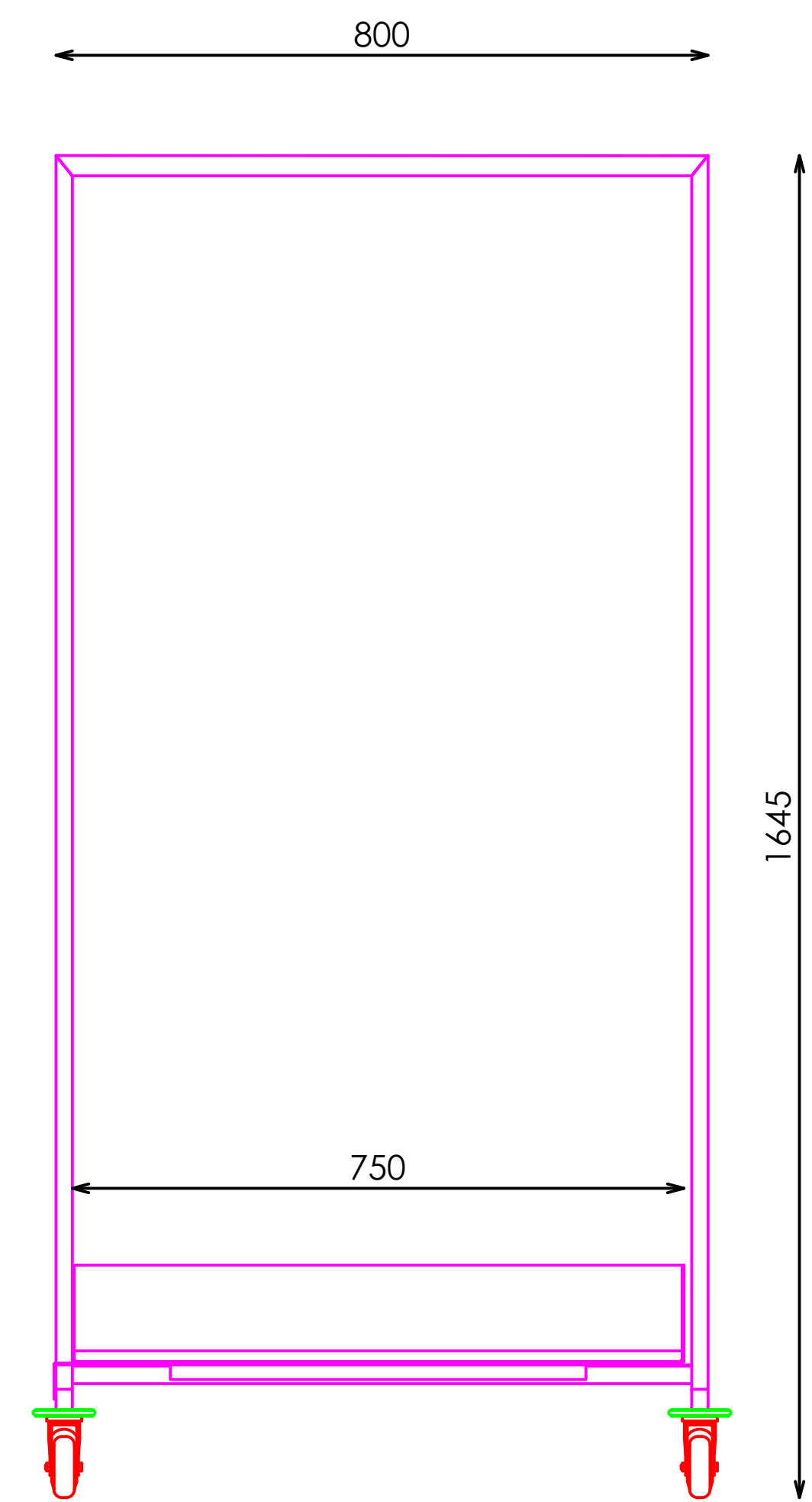
ALZADO FRONTAL
