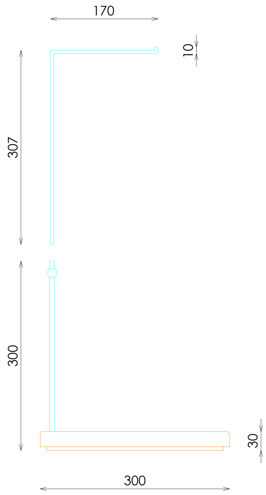
ALZADO
