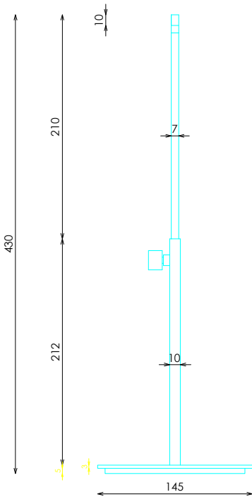
ALZADO
